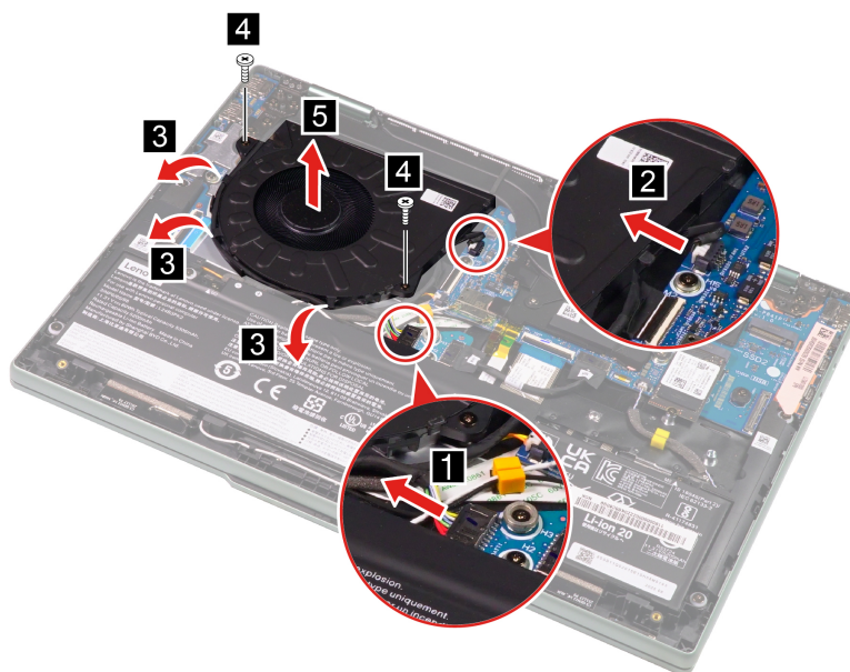
Figure 12. Remove the fan
