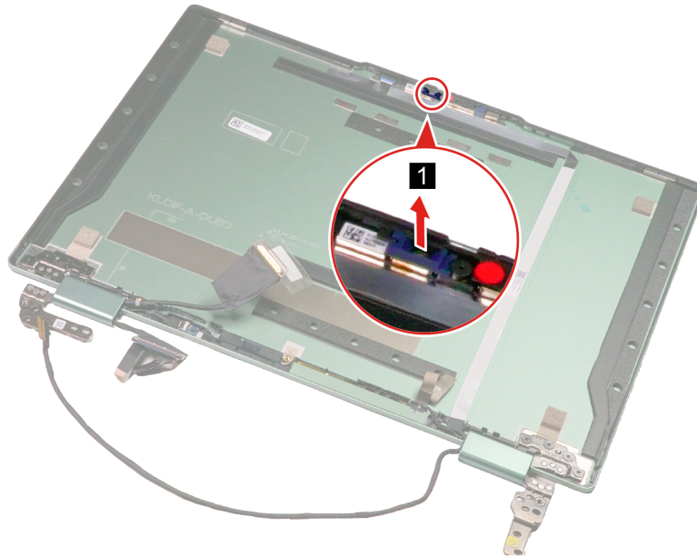
Figure 27. Remove the IR rubber
