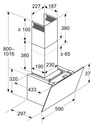
Maße in mm Gerät im Umluftbetrieb
