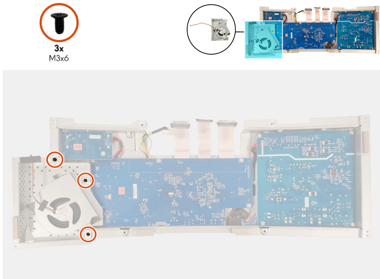
Figure 24. Installing the fan module
