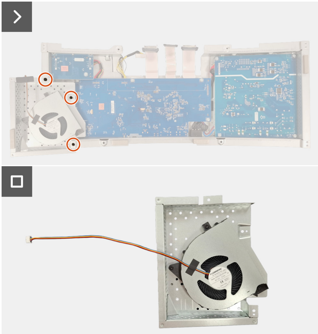
Figure 23. Removing the fan module
