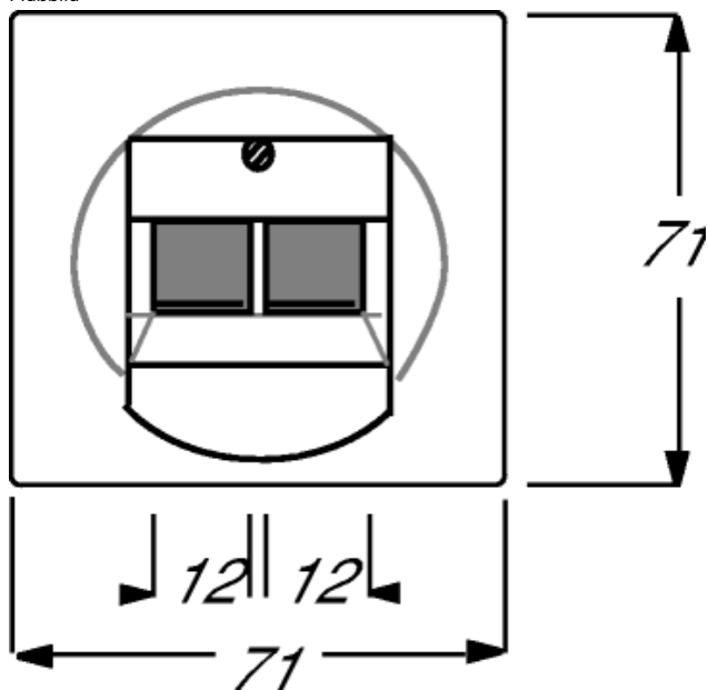
Maßbild
