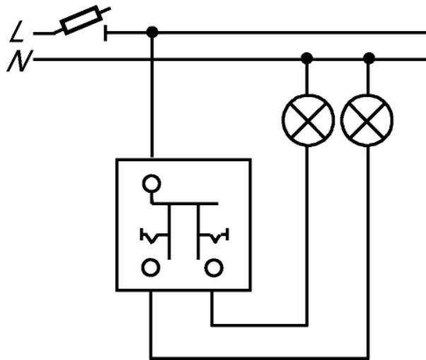
Anschlussbild
