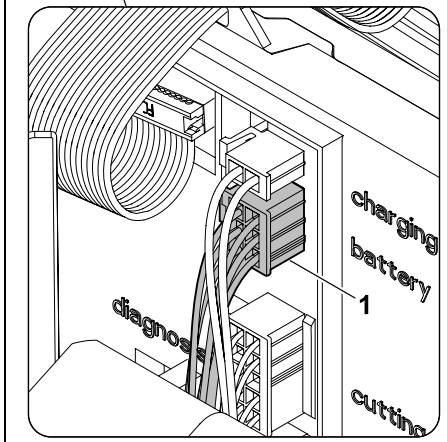
Kabelstecker (1) (battery) abziehen.
