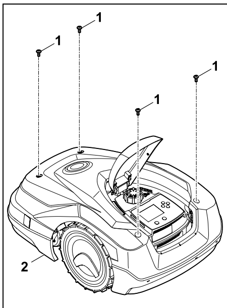
Wykręcić śruby (1) na osłonie (2) i wyjąć. Wyciągnąć osłonę (2) do góry.
