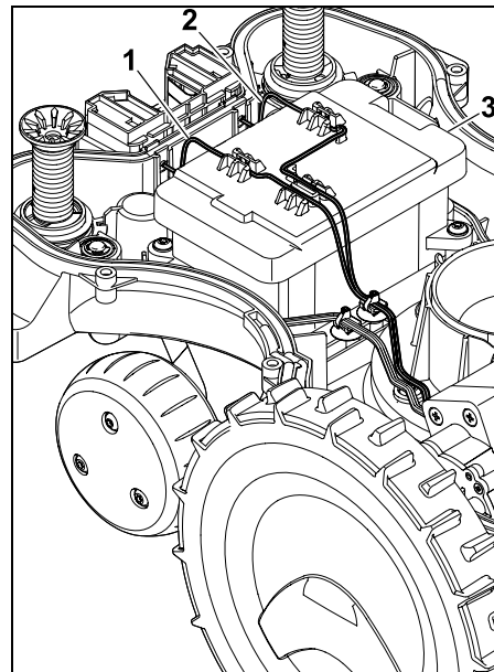
Kabel (1) und Kabel (2) aus den Kabelführungen entnehmen und Akku (3) entnehmen.
