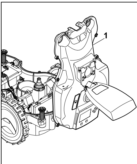
Gehäuseoberteil (1) nach hinten aufklappen.
