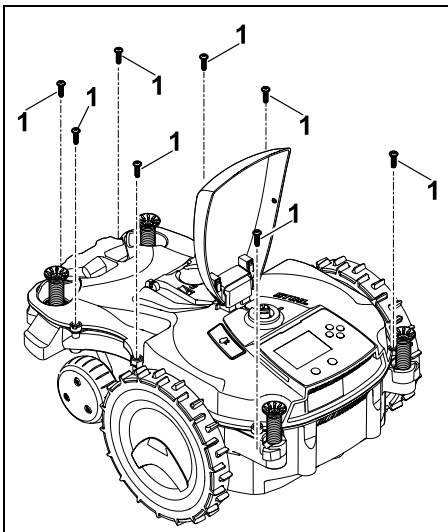
Schrauben (1) ausdrehen und entnehmen.
