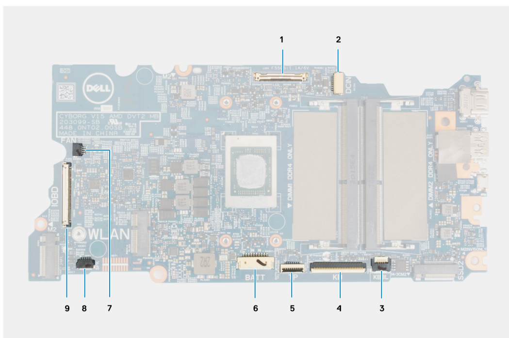
Abbildung 1. Systemplatinenanschlüsse
