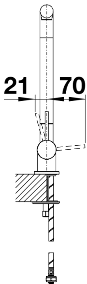
Seitenansicht Hebel 2D
