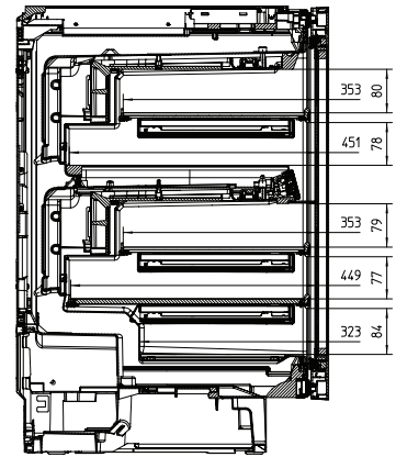
KWT6322UG, KWT6322UG edt/cs, Innenraummaße (Skizze)
