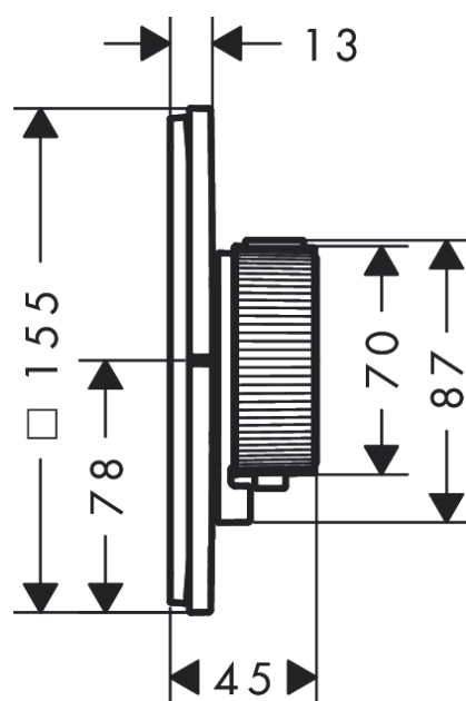
Maßzeichnung
