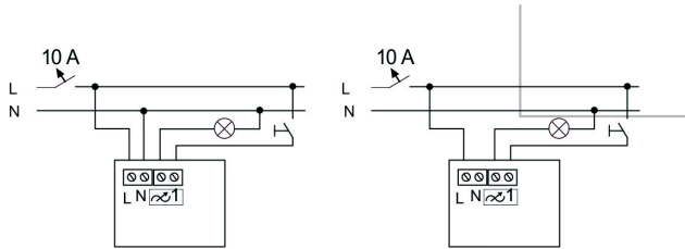
Anschlussbild
