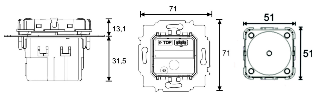
Maßbild
