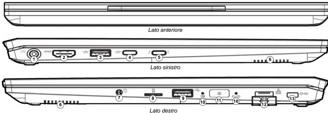
Figura 3 - Vista anteriore, sinistra e destra (Modello A)
