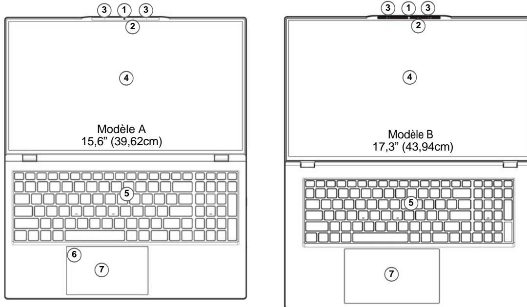
Figure 2 - Vue de face avec l'écran ouvert
