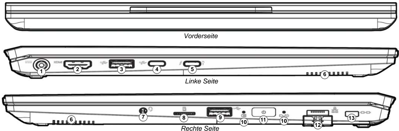
Abb. 3 - Ansicht von vorne, links und rechts (Modell A)
