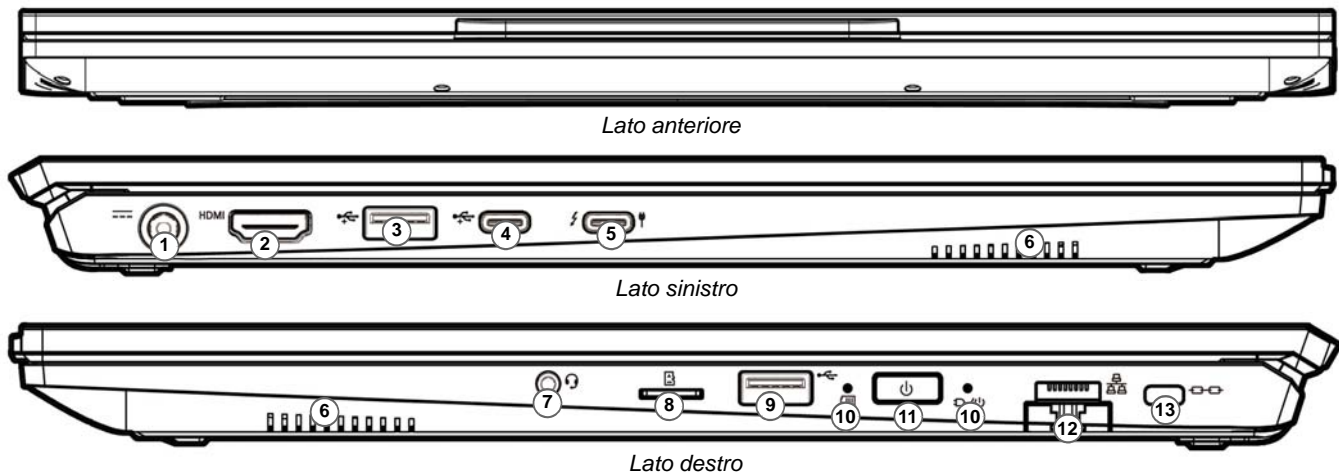
Figura 4 - Vista anteriore, sinistra e destra (Modello B)
