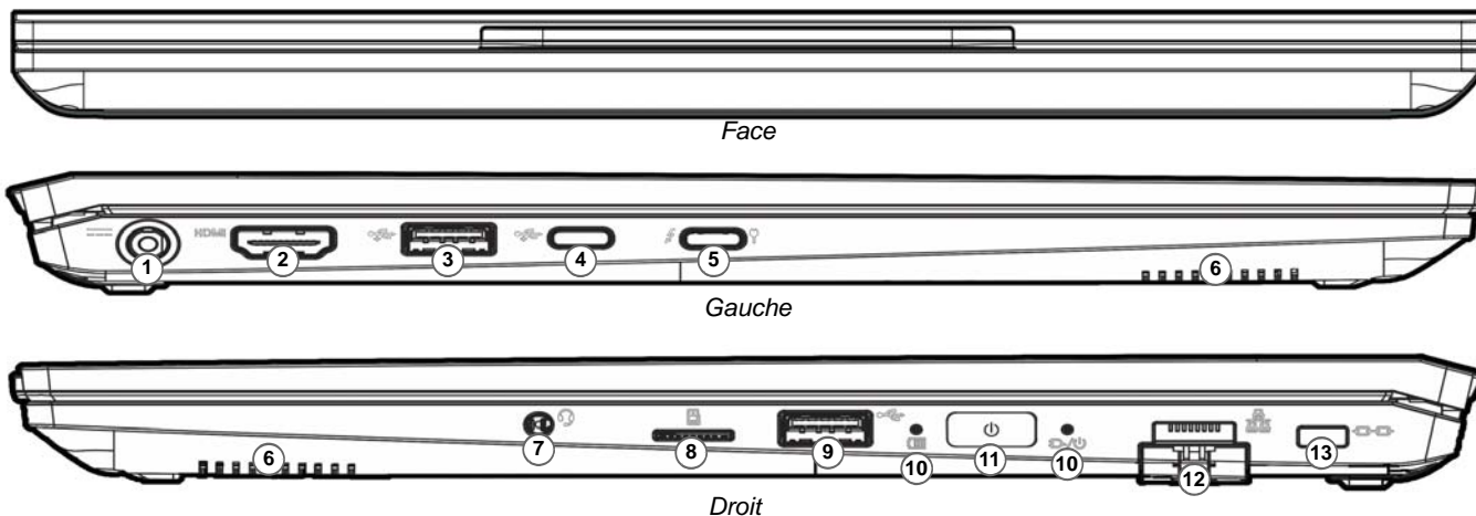
Figure 3 - Vues de face, gauche et droite (Modèle A)
