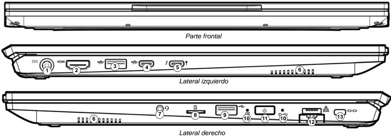
Figura 4 - Vistas frontal, izquierda y derecha (Modelo B)
