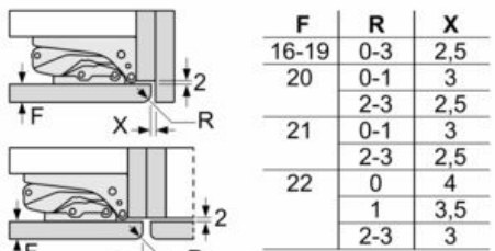
Maße in mm Empfehlung Spaltmaße für Flachscharnier
