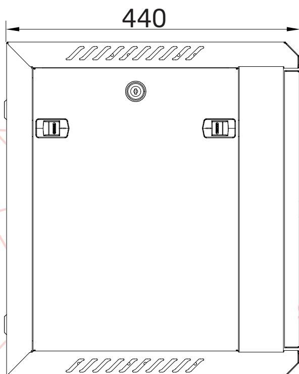
Seitenansicht
