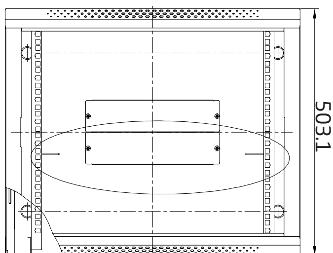
Vorderseiteninnenansicht
