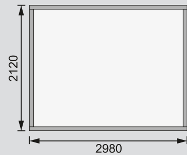
Fundamentplan ohne Boden (in mm)
