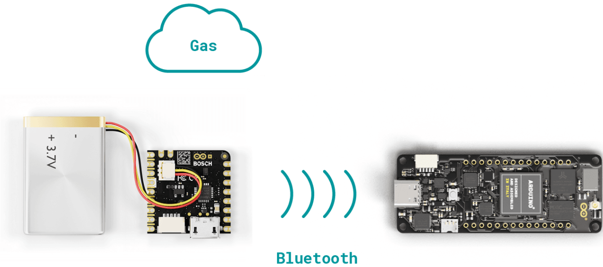
远程环境监测的典型解决方案示例，包括Arduino® Nicla Sense ME、Portenta H7和电池。请注意电池电缆在电路板连接器中的方向。
