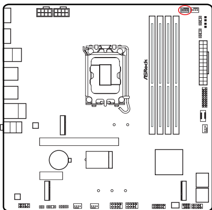
CPU_FAN1
