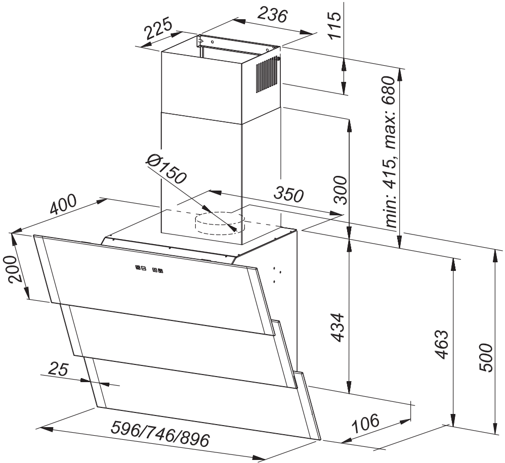
Abb. 18 Abmessungen Modelle „Lito“
