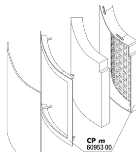
JBL CristalProfi m greenline Halterung FilterPad
