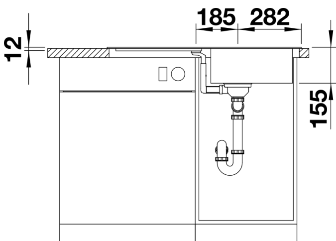
Frontansicht
