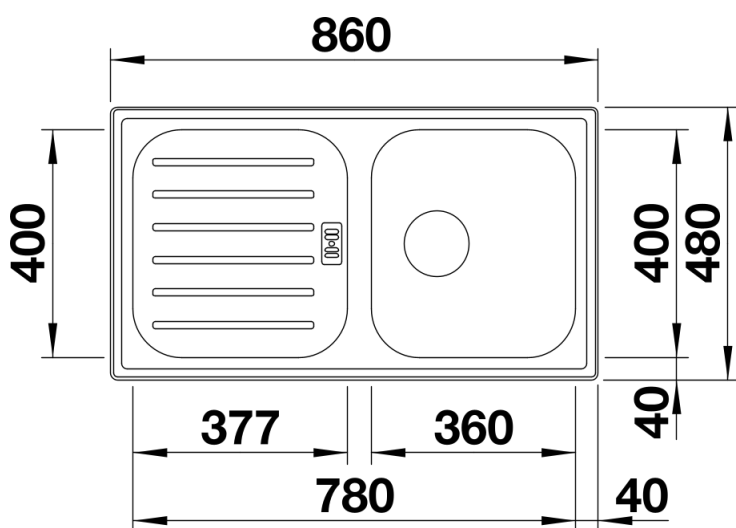
Aufsicht
