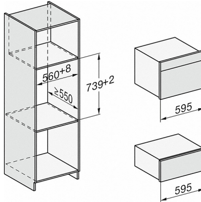
ESW7x20, Skizze
