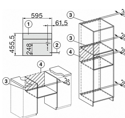
DGC7x40, Skizze
