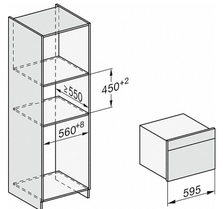
DGC7x4x, DGC7x4xX Skizze
