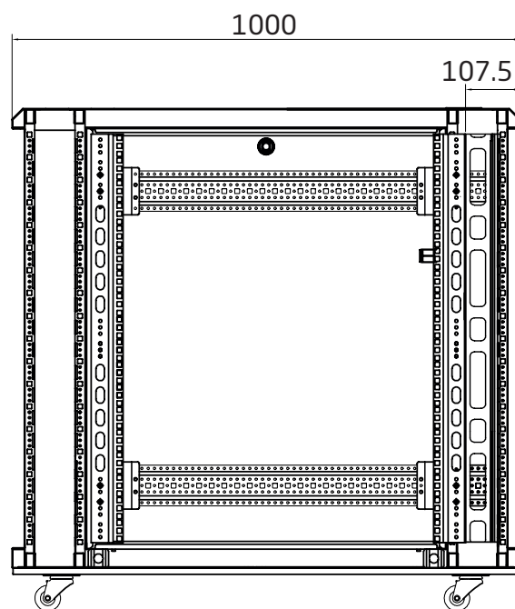
Seiteninnenansicht
