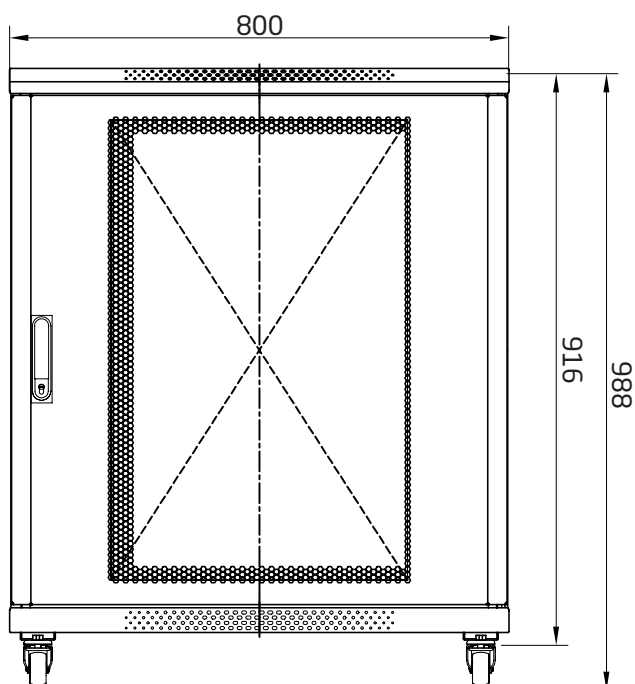
Hinteransicht
