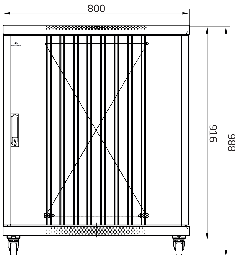
Vorderansicht
