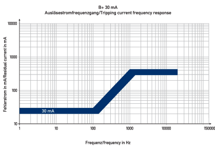
Kennlinie B+ 30 mA
