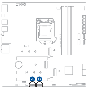
A USB_E34
