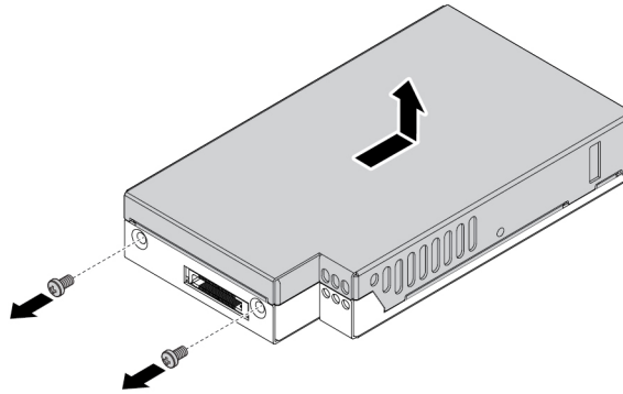
Abbildung 59. Entfernen der Abdeckung vom Träger des M.2-Solid-State-Laufwerks
