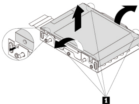
Abbildung 53. Speicherlaufwerk aus dem Adapter entfernen
