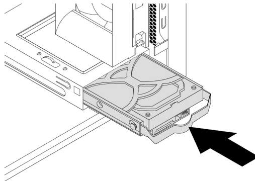
Abbildung 99. Sekundäres Speicherlaufwerk installieren
