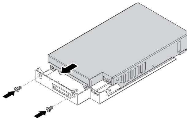
Abbildung 62. Installieren der Abdeckung am Träger des M.2-Solid-State-Laufwerks
