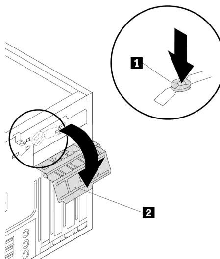
Abbildung 25. PCIe-Kartenverriegelung öffnen
