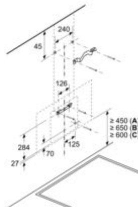
Maße in mm Wandinstallation mit Kamin
