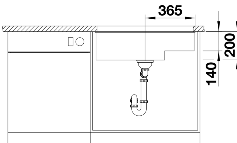
Frontansicht
