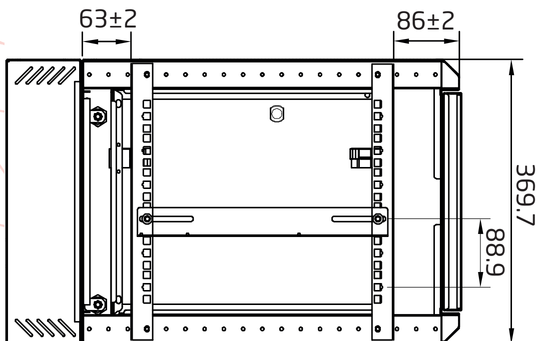
Seiteninnenansicht
