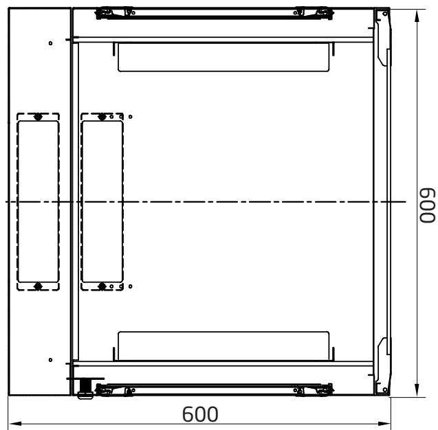
Boden
