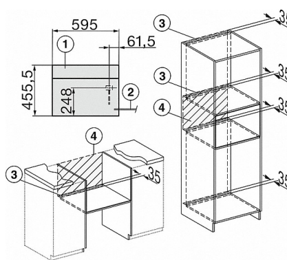
DGC7x40, Skizze
