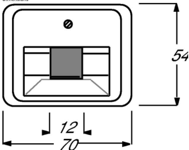
Dimensions
