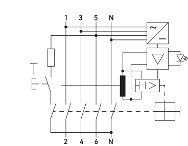
Anschlussschema
