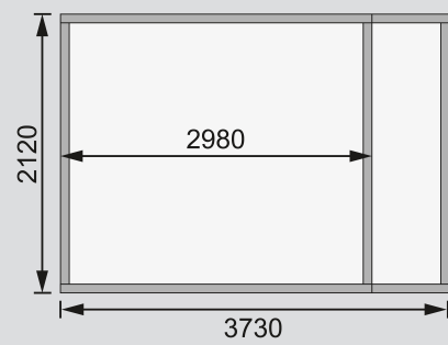
Fundamentplan ohne Boden (in mm)
