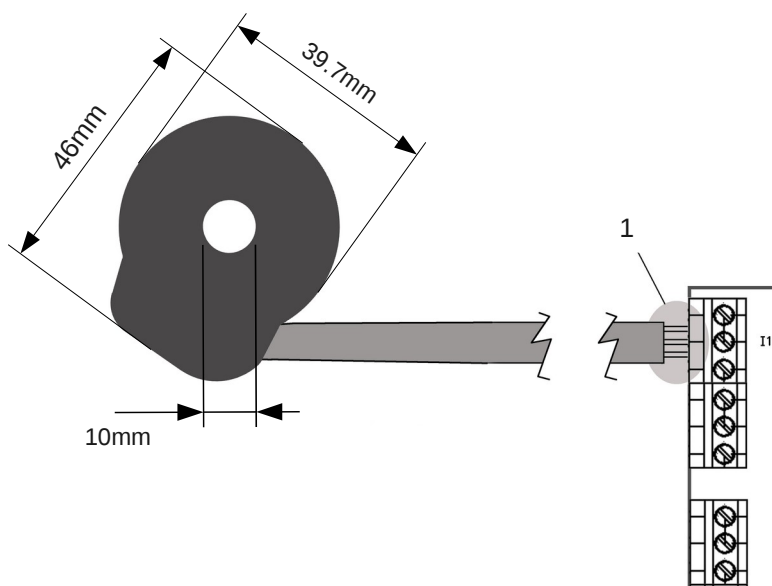
Abbildung 2: Maße des 85A Stromsensors in mm
