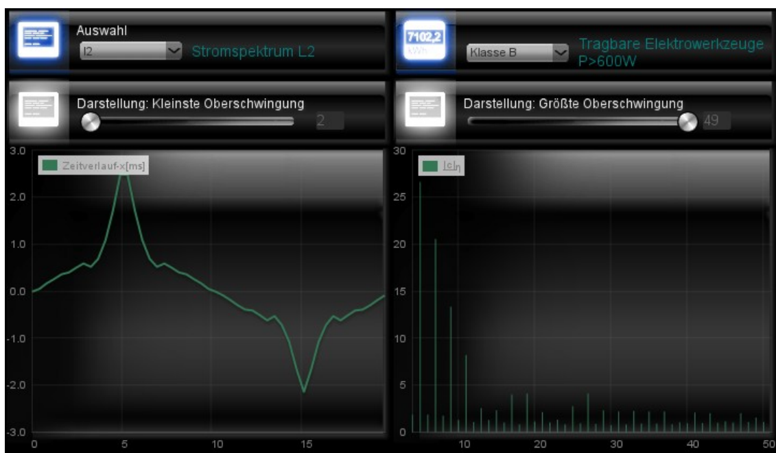
Abbildung 25: Visualisierung Oberschwingungen
