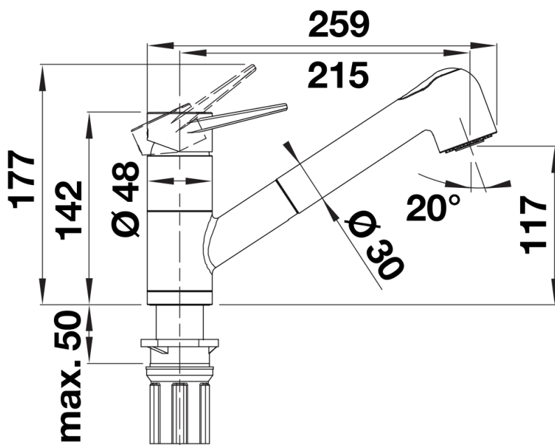
Seitenansicht
