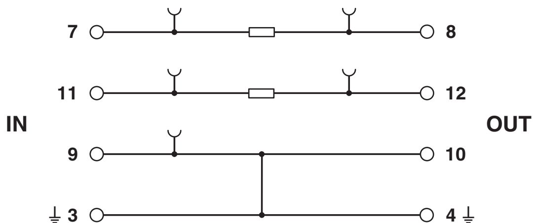
Schaltplan
