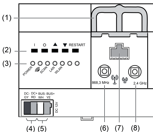
Bild 1: Frontansicht eNet Server
