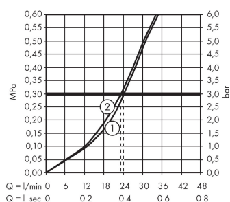
Durchflussdiagramm
