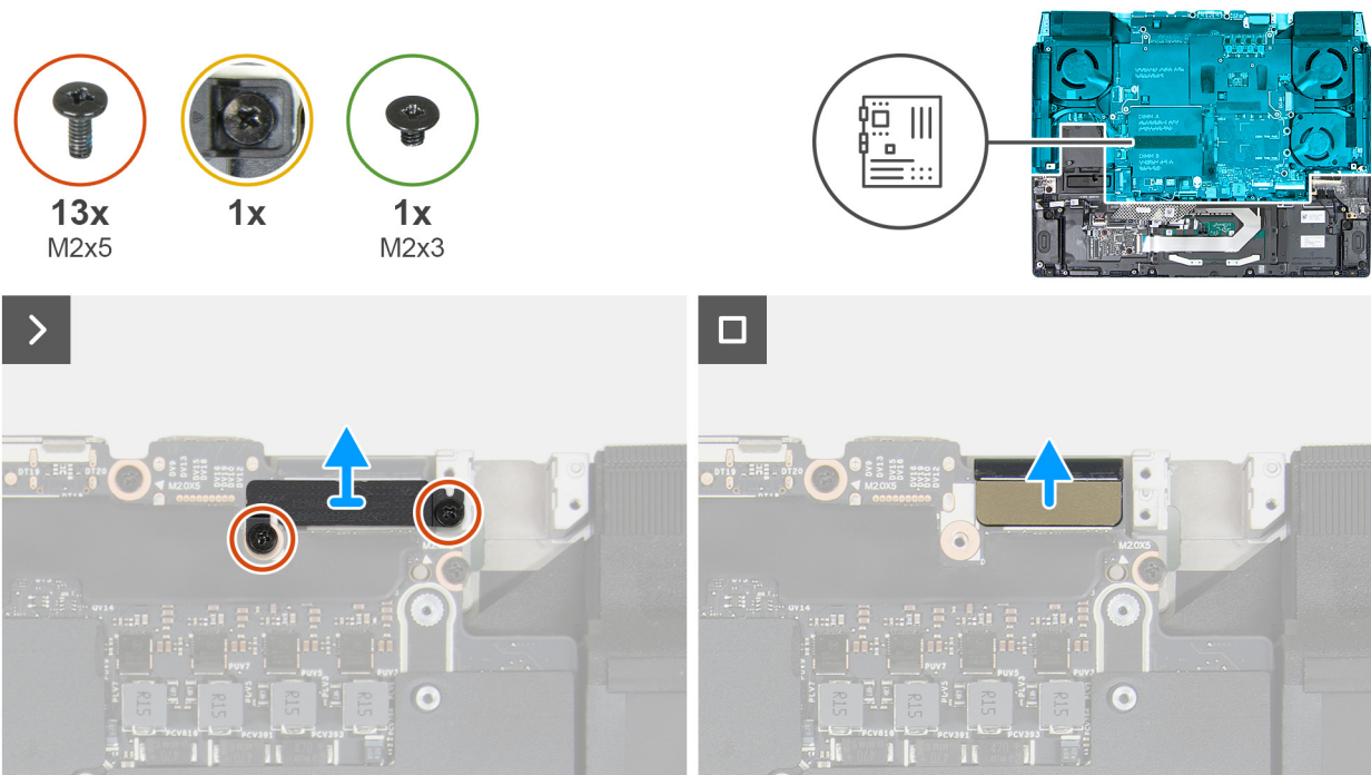
Abbildung 56. Entfernen des Bildschirmkabels
