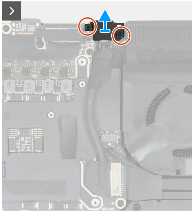
Abbildung 53. Entfernen des Netzadapteranschlusses
