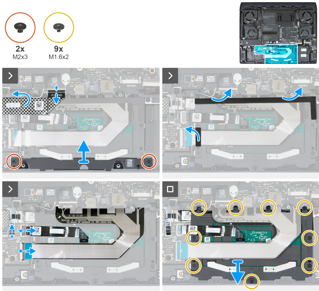
Abbildung 34. Entfernen der Touchpad-Baugruppe
