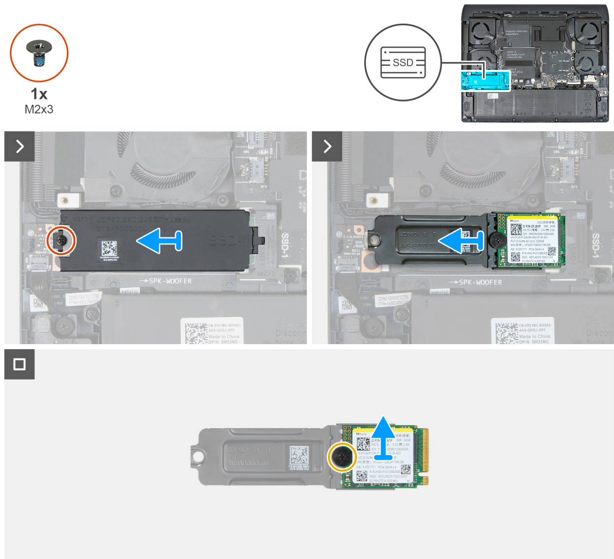
Abbildung 22. Entfernen des M.2-2230-SSD aus Steckplatz 1
