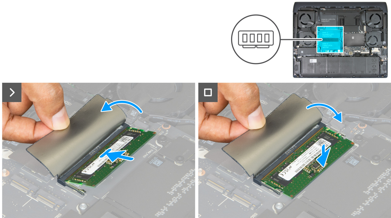
Abbildung 21. Wiedereinbauen des Speichermoduls
