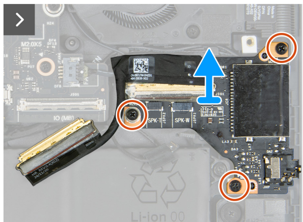
Abbildung 32. Entfernen der I/O-Platine
