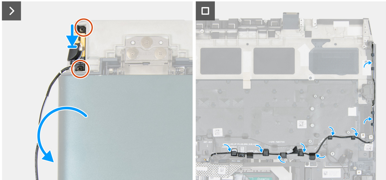
Abbildung 74. Einbauen der WLAN-Hauptantenne
