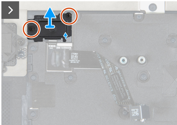
Abbildung 71. Entfernen des Netzschalters
