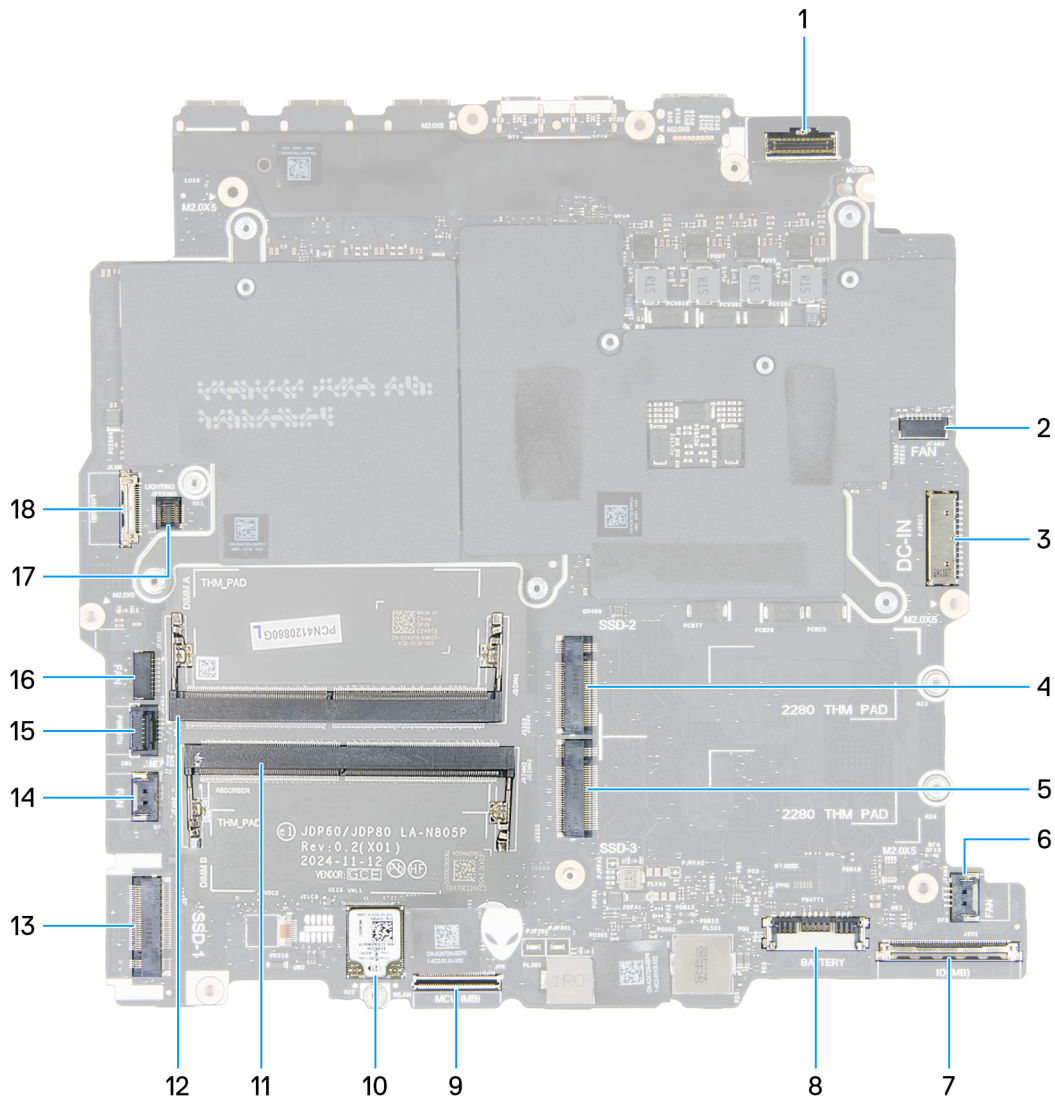
Abbildung 63. Anschlüsse auf der Hauptplatine
