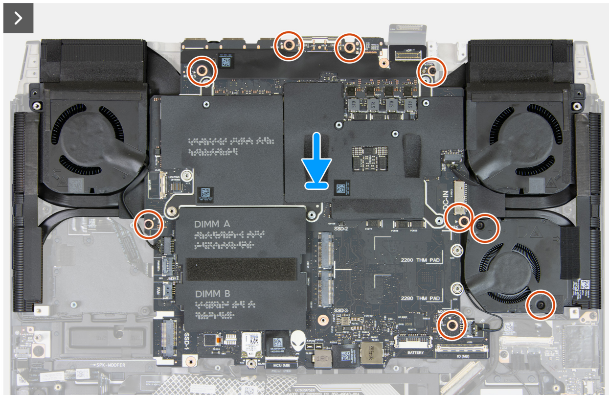
Abbildung 64. Einbauen der Systemplatine
