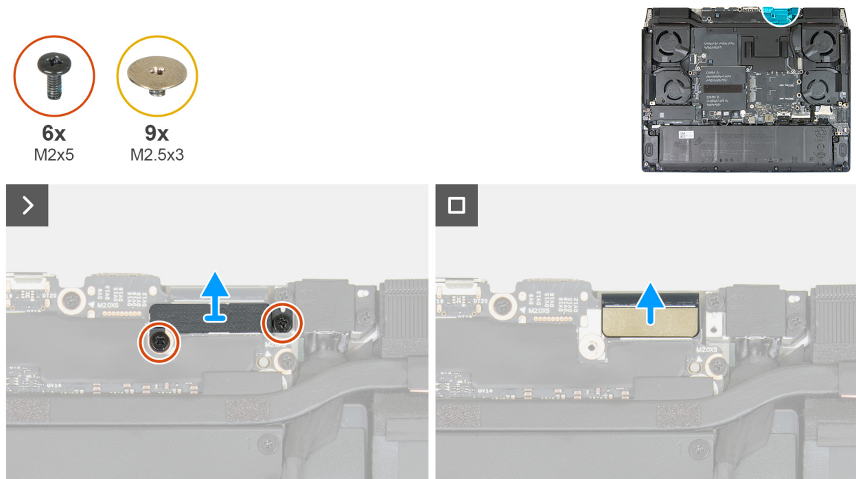
Abbildung 46. Entfernen der Bildschirmbaugruppe
