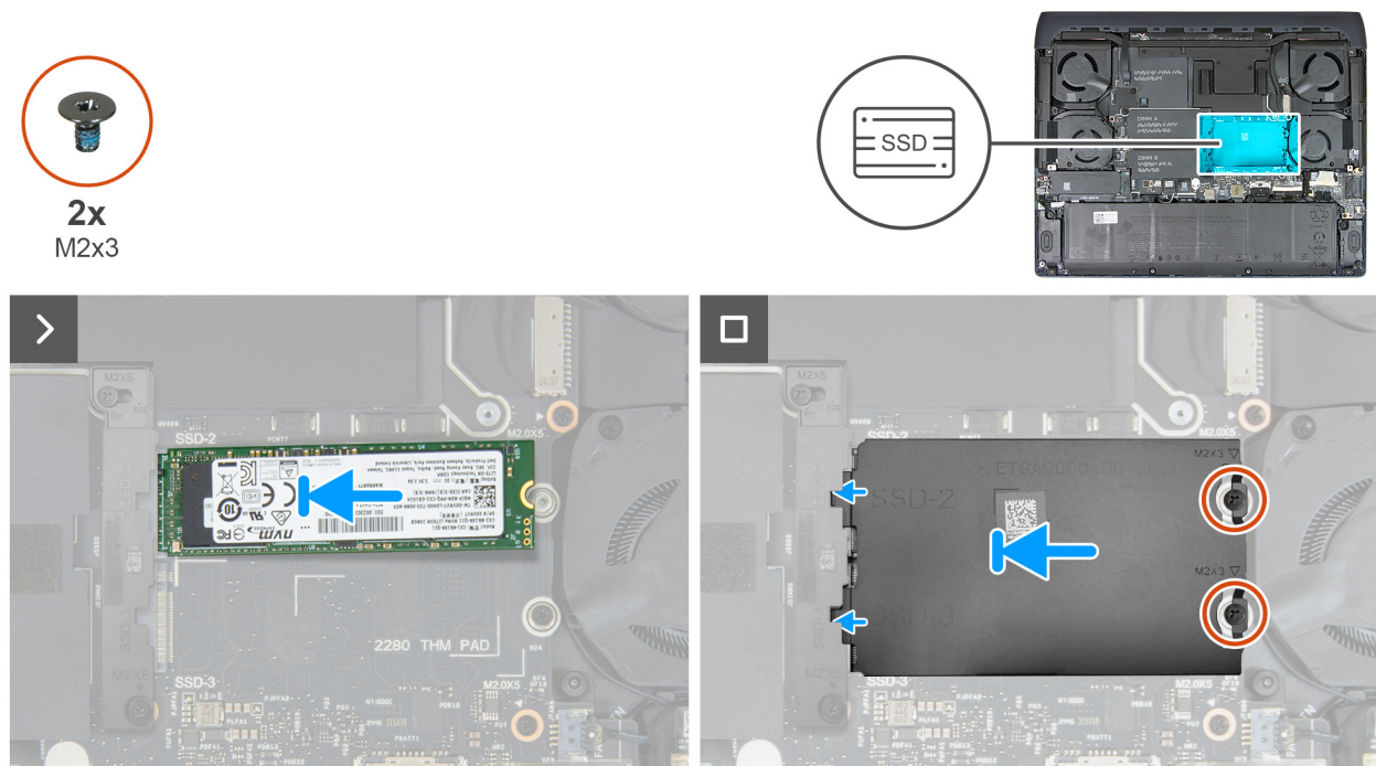
Abbildung 27. Installieren des M.2-2280-SSD in Steckplatz 2 und Steckplatz 3
