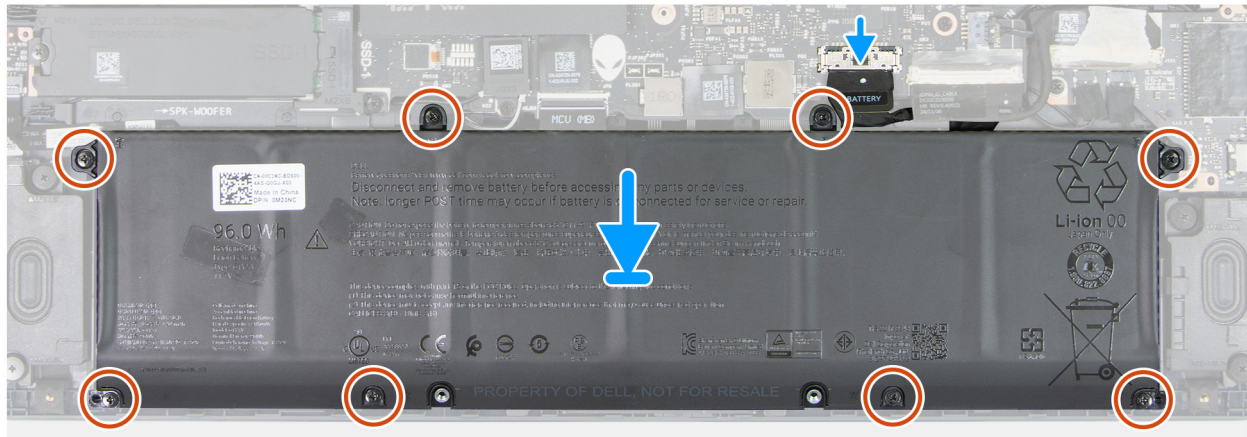
Abbildung 17. Wiedereinbauen des Akkus
