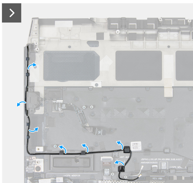
Abbildung 75. Entfernen der WLAN-Aux-Antenne
