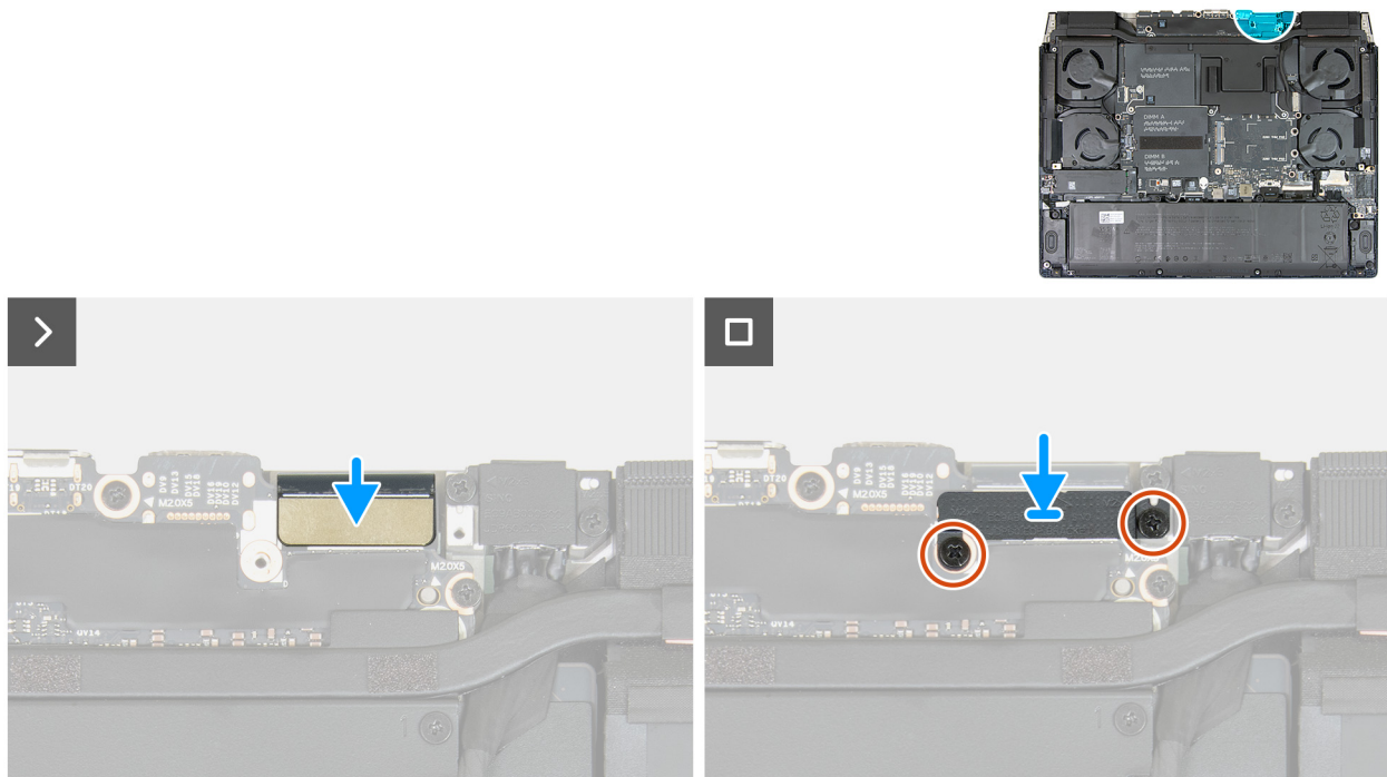
Abbildung 51. Einbauen der Displaybaugruppe
