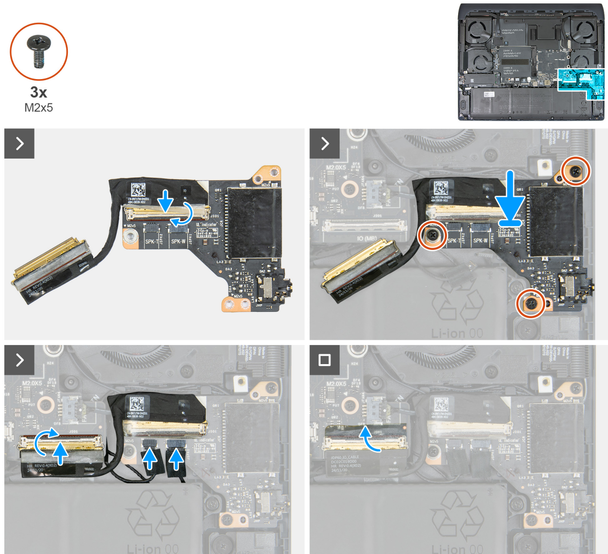
Abbildung 33. Installieren der I/O-Platine
