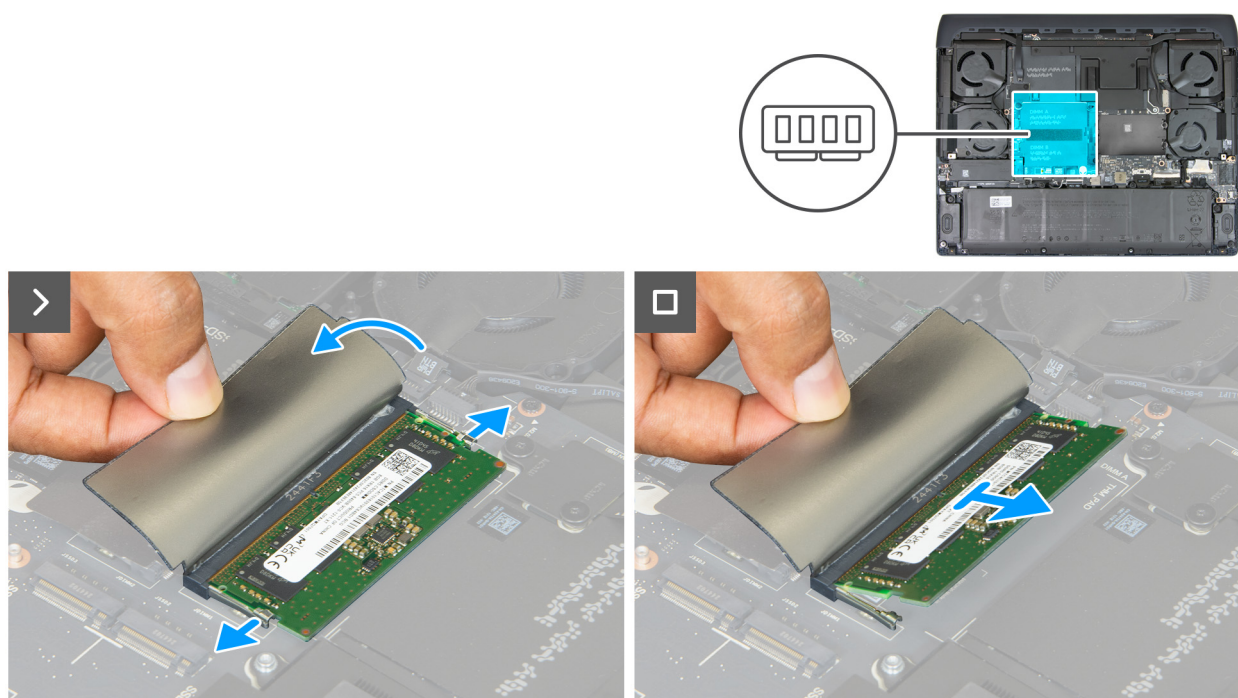
Abbildung 20. Entfernen des Arbeitsspeichermoduls
