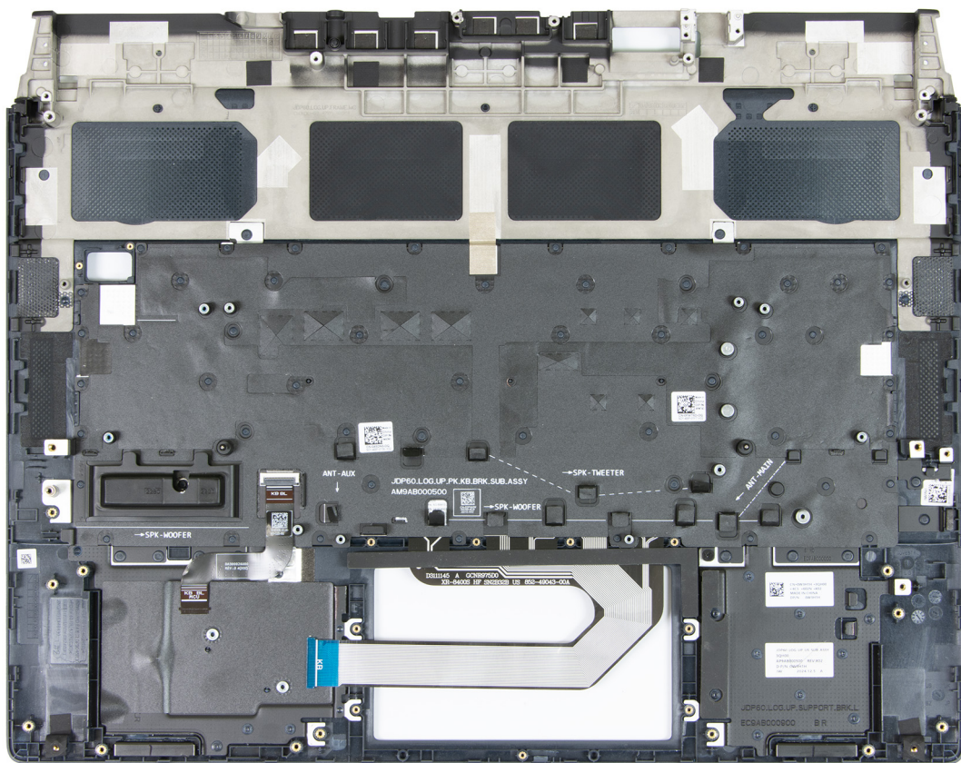
Abbildung 80. Entfernen der Handballenstützen- und Tastaturbaugruppe
