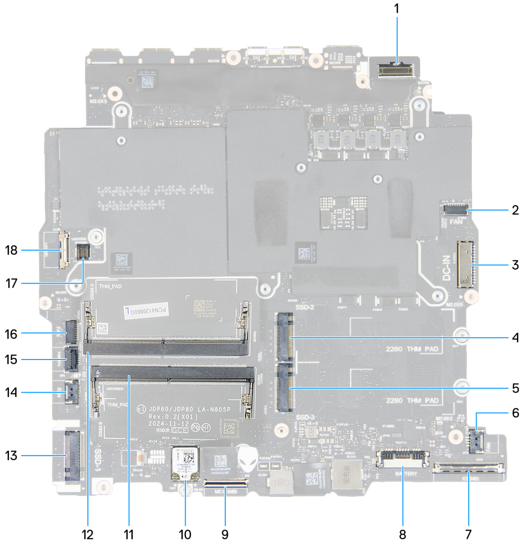
Abbildung 55. Anschlüsse auf der Hauptplatine
