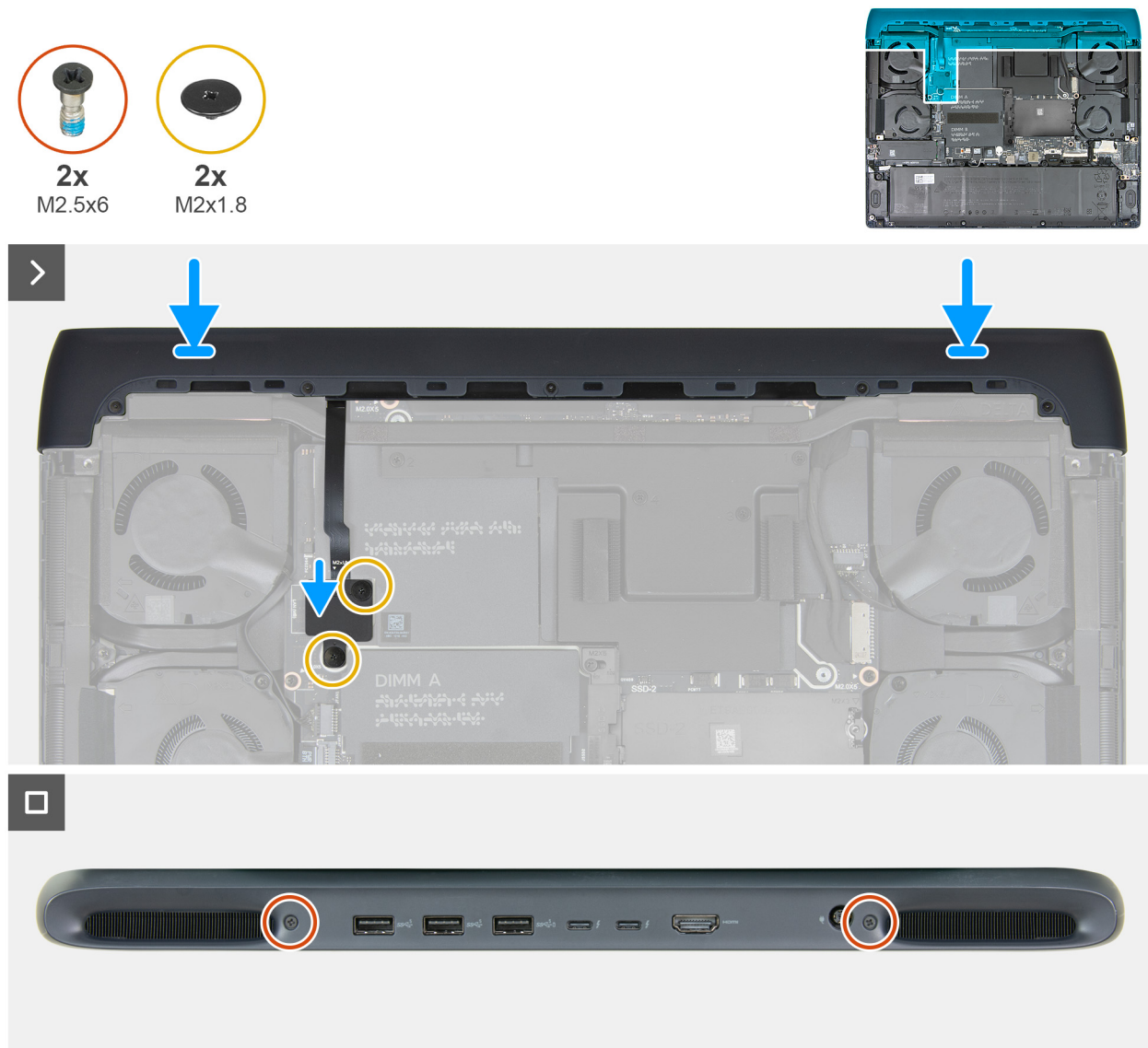
Abbildung 29. Einbauen der I/O-Abdeckung
