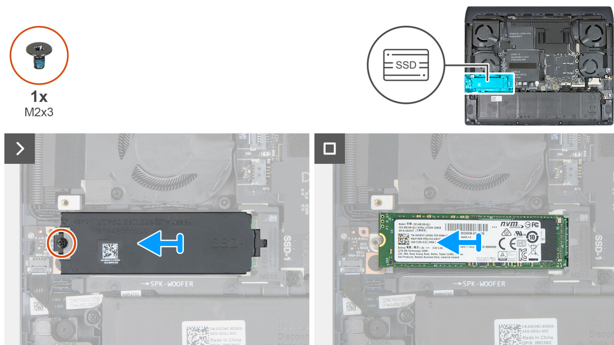
Abbildung 24. Entfernen des M.2-2280-SSD aus Steckplatz 1
