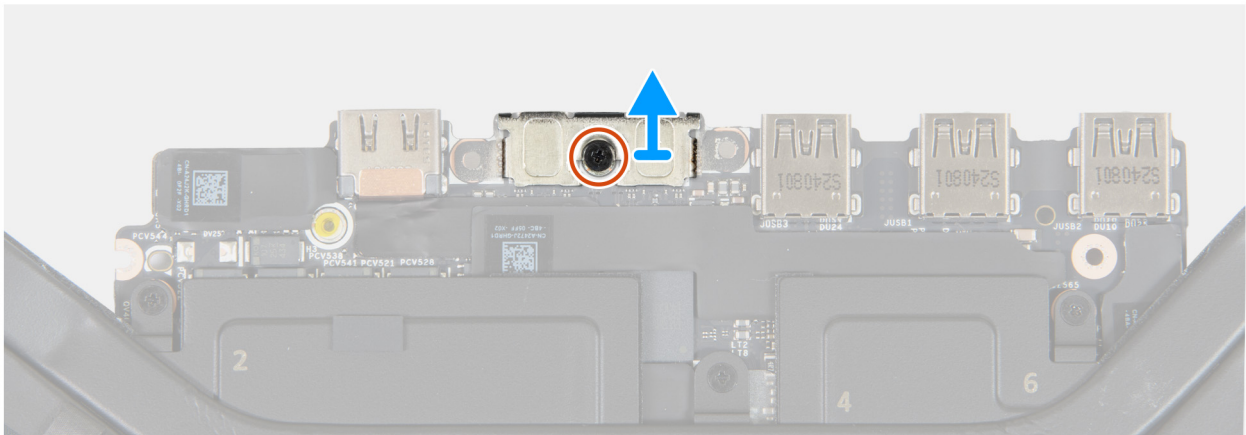
Abbildung 59. Entfernen der USB-Typ-C-Halterung
