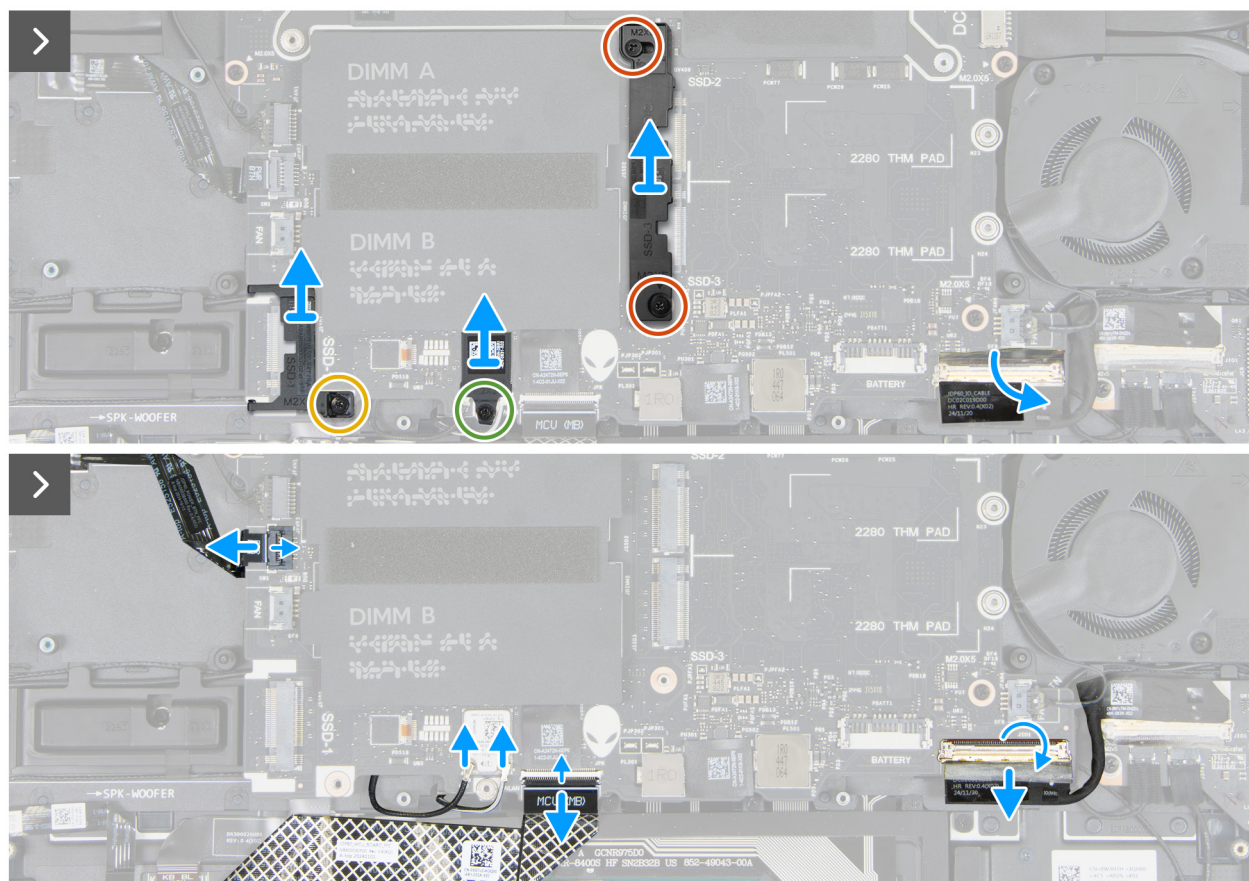
Abbildung 57. Trennen der Kabel von der Hauptplatine
