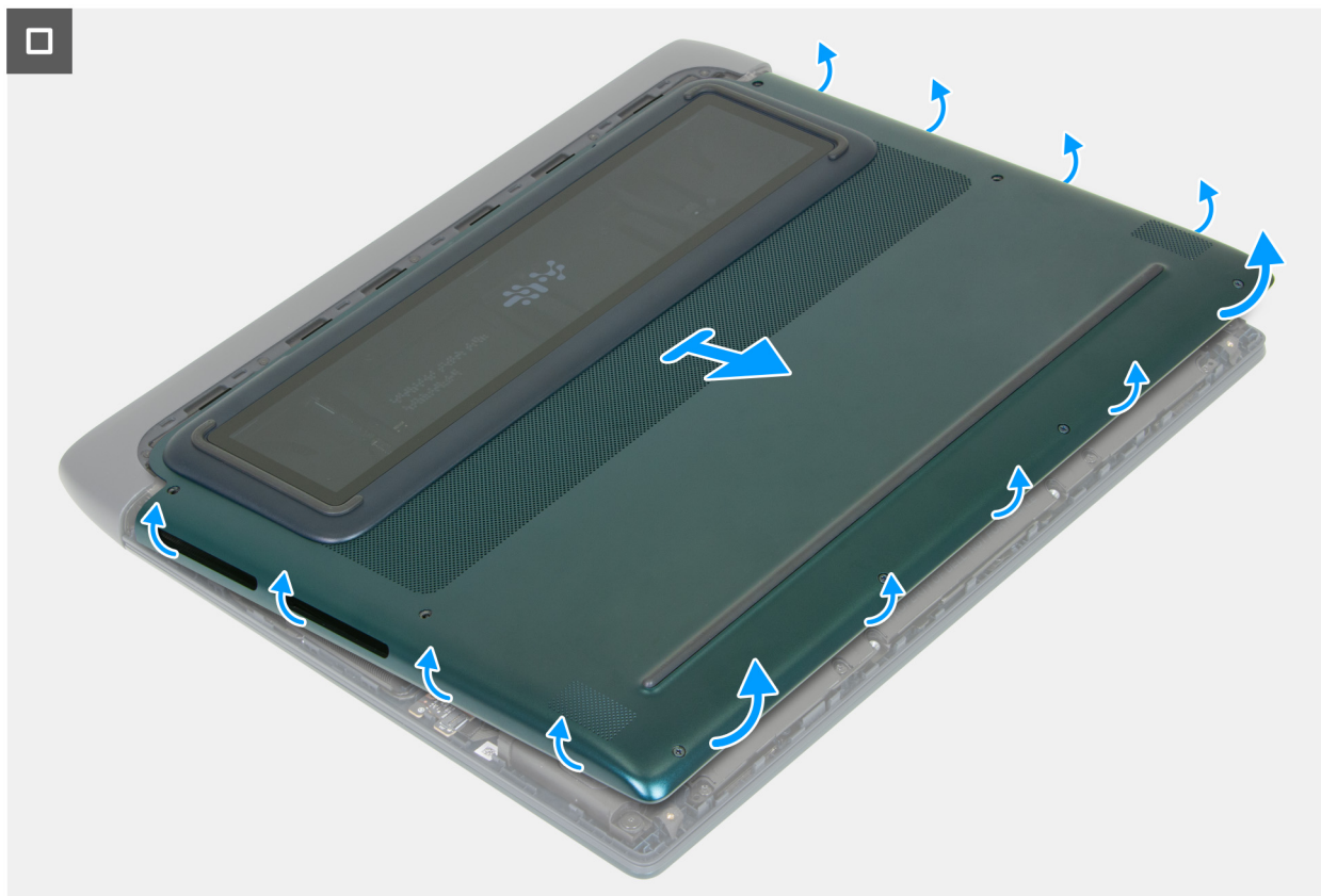
Abbildung 11. Anheben der Bodenabdeckung
