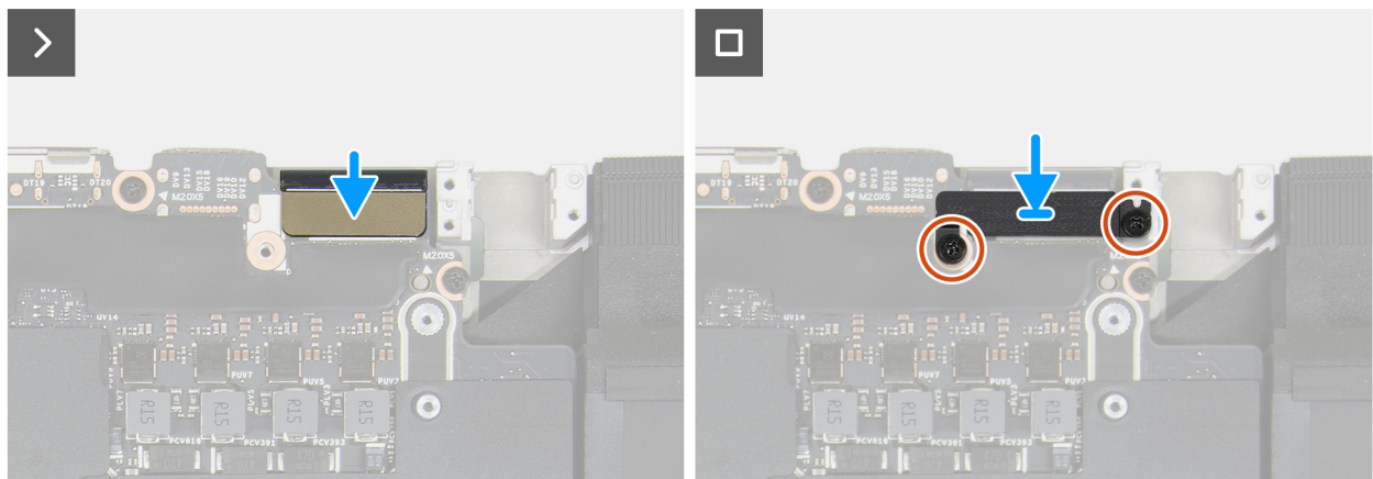
Abbildung 66. Einbauen der Bildschirmkabelhalterung
