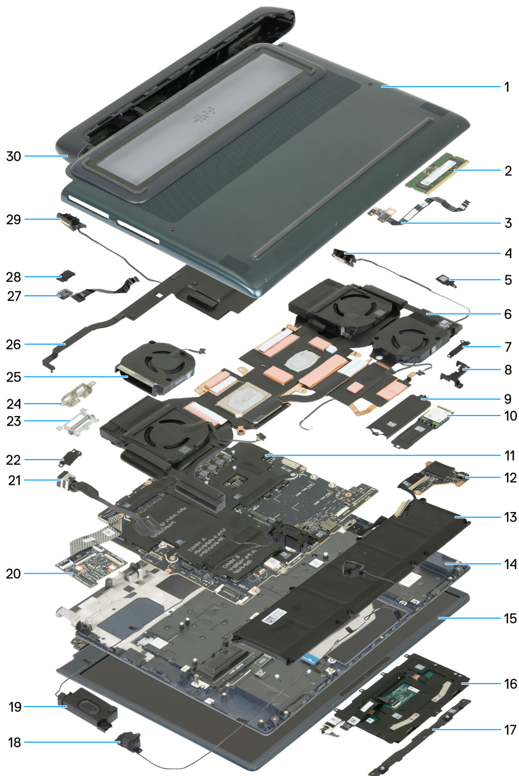
Abbildung 9. Hauptkomponenten des Alienware 16 Area-51 AA16250
