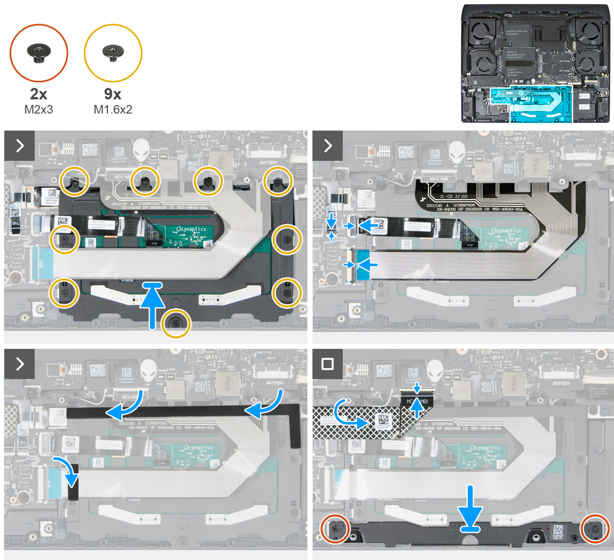
Abbildung 37. Installieren der Touchpad-Baugruppe
