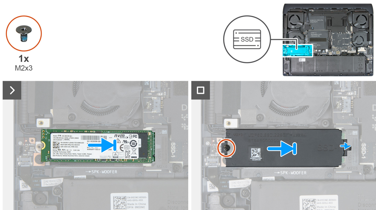
Abbildung 25. M.2-2280-SSD in Steckplatz 1 erneut anbringen
