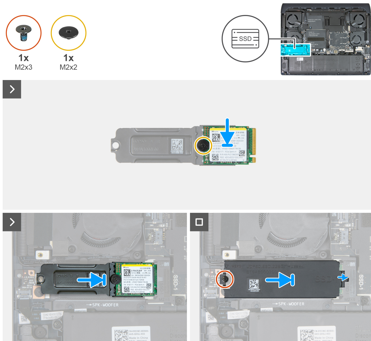
Abbildung 23. Installieren der M.2-2230-SSD in Steckplatz 1
