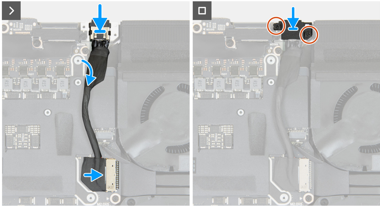
Abbildung 54. Einbauen des Netzadapteranschlusses
