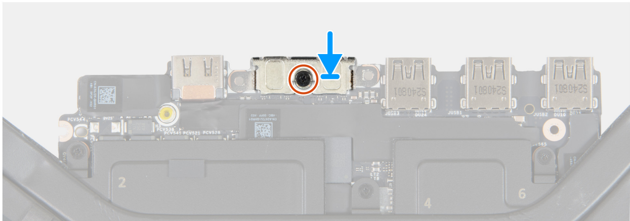
Abbildung 67. Einbauen der USB-Typ-C-Halterung
