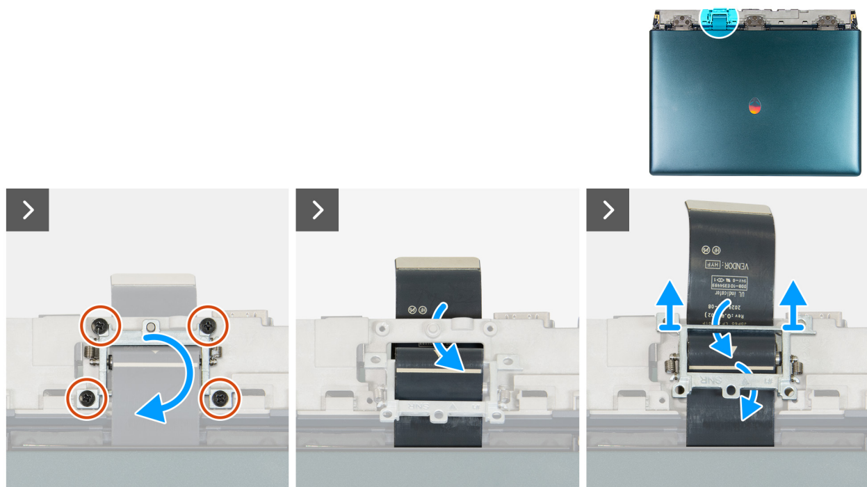
Abbildung 47. Entfernen der Bildschirmbaugruppe
