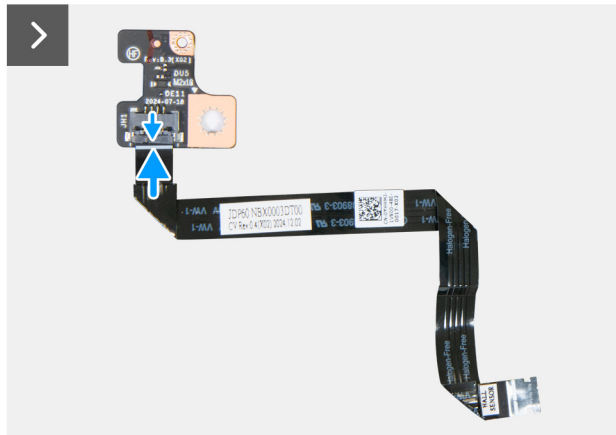
Abbildung 43. Installieren der Hall-Sensorplatine
