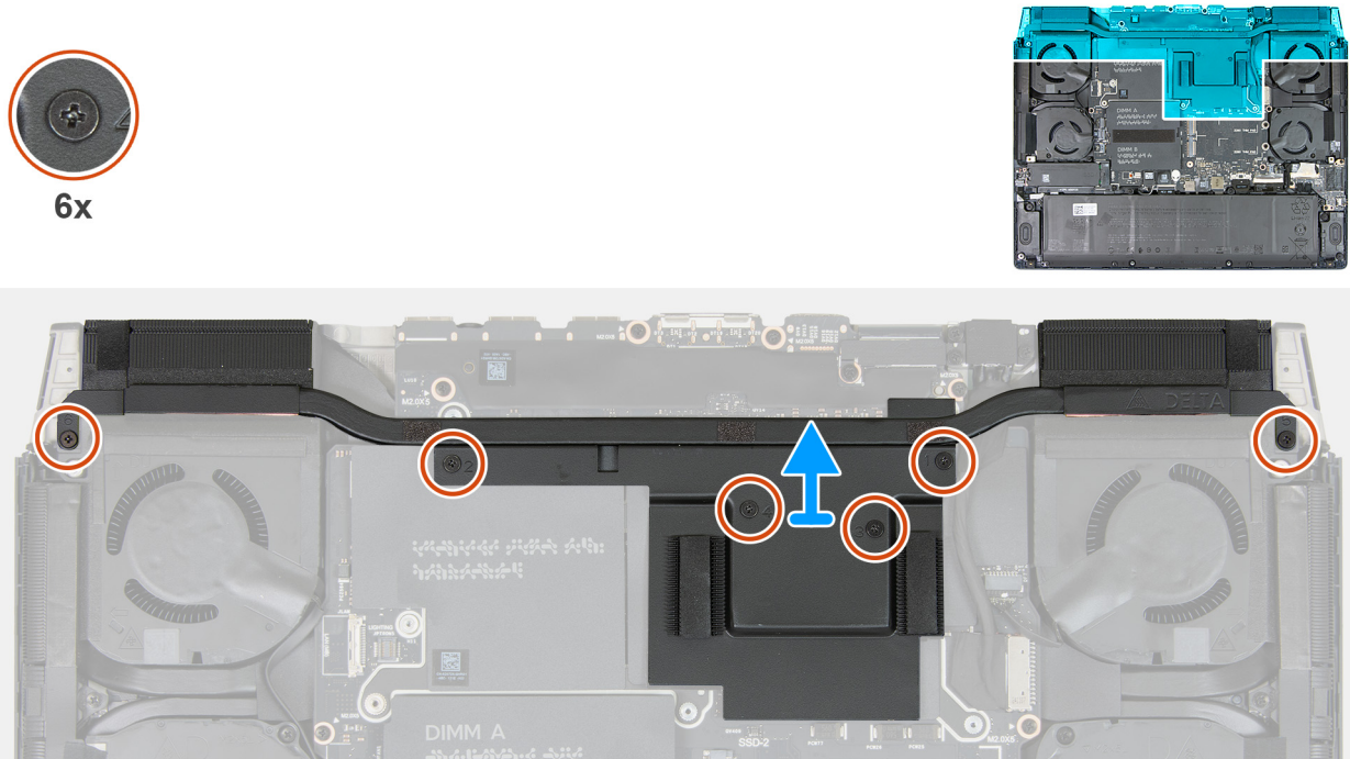
Abbildung 44. Entfernen des VR-Kühlkörpers
