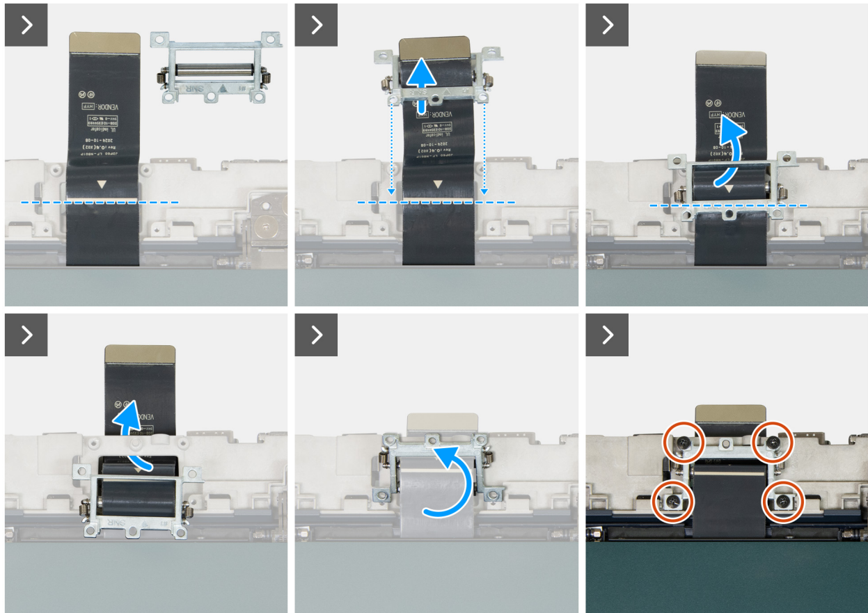
Abbildung 50. Einbauen der Displaybaugruppe
