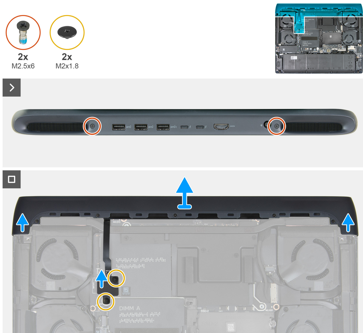
Abbildung 28. Entfernen der hinteren E/A-Abdeckung
