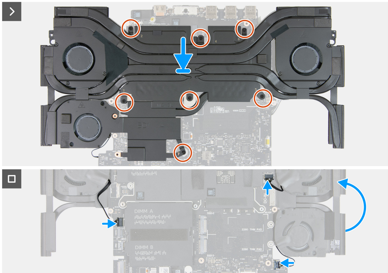
Abbildung 70. Installieren der Lüfter- und Kühlkörperbaugruppe
