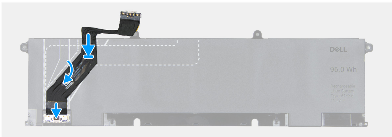
Abbildung 19. Einsetzen des Akkukabels
