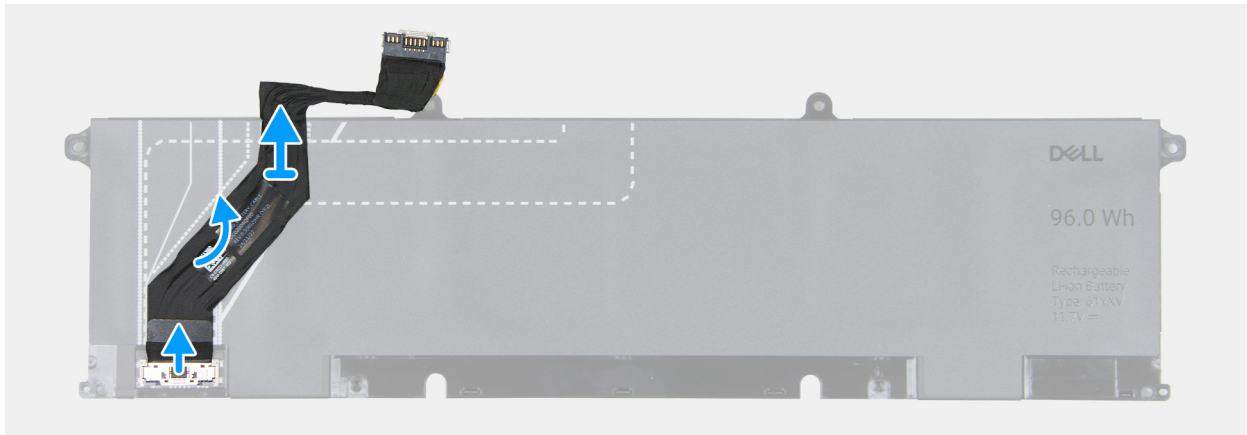
Abbildung 18. Entfernen des Akkukabels
