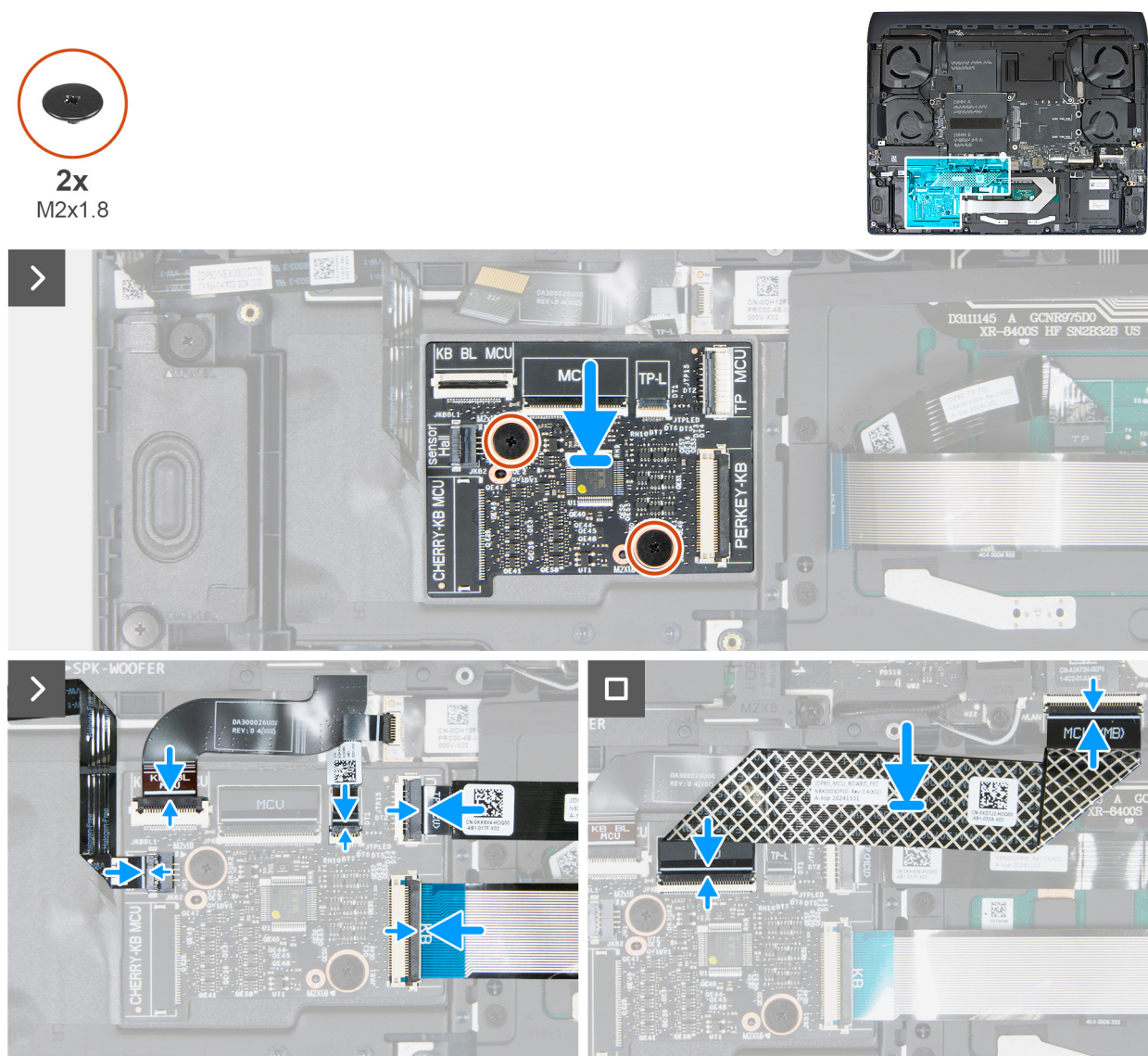
Abbildung 41. Installieren der Tastatursteuerungsplatine
