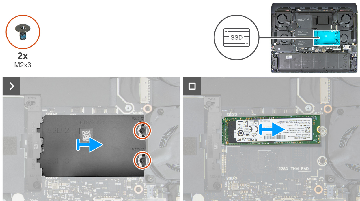
Abbildung 26. Entfernen des M.2-2280-SSD aus Steckplatz 2 und Steckplatz 3
