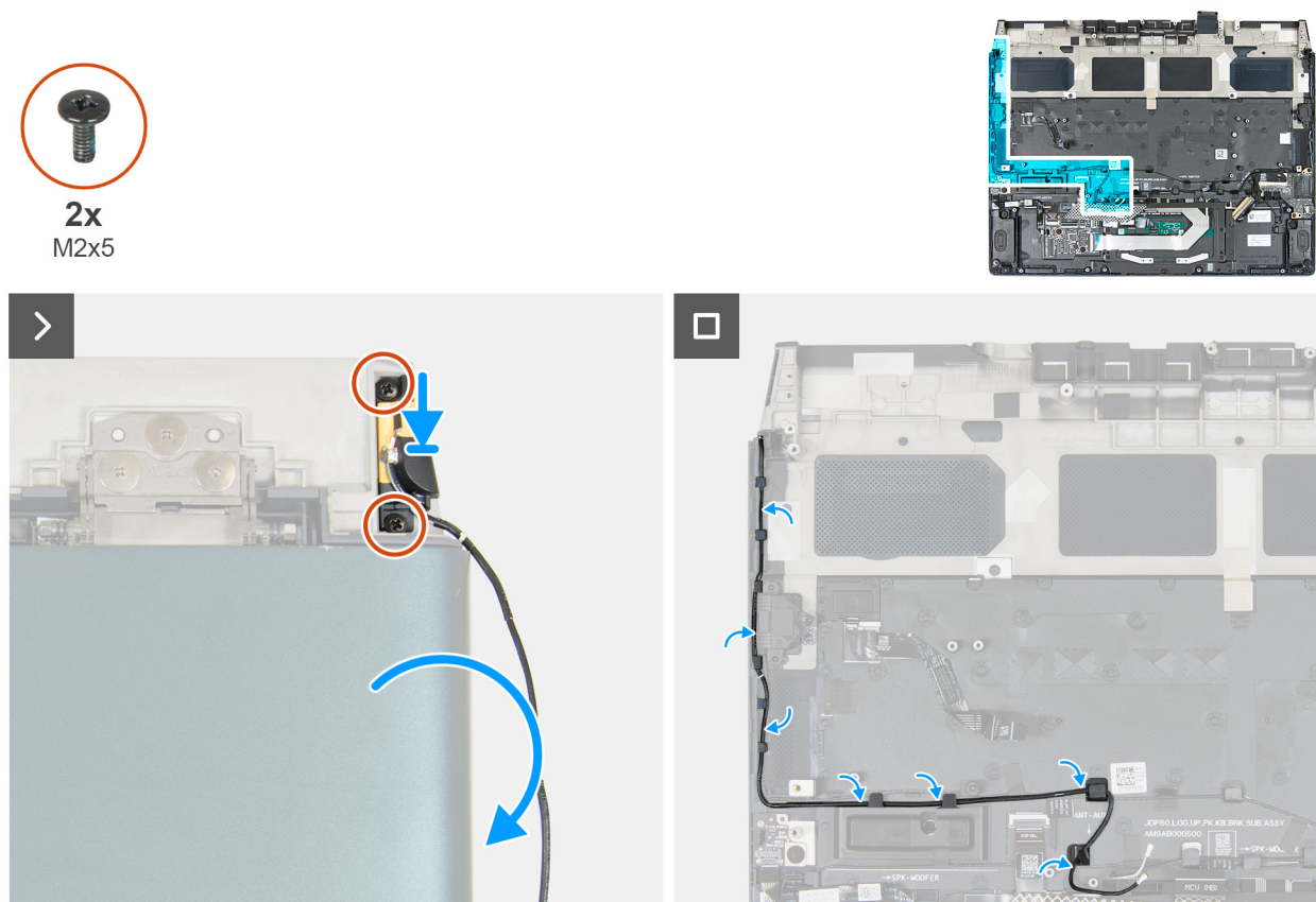
Abbildung 76. Installieren der WLAN-Aux-Antenne
