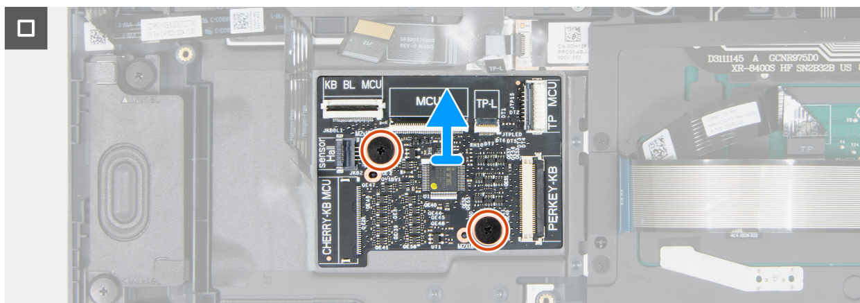
Abbildung 40. Entfernen der Tastatursteuerungsplatine
