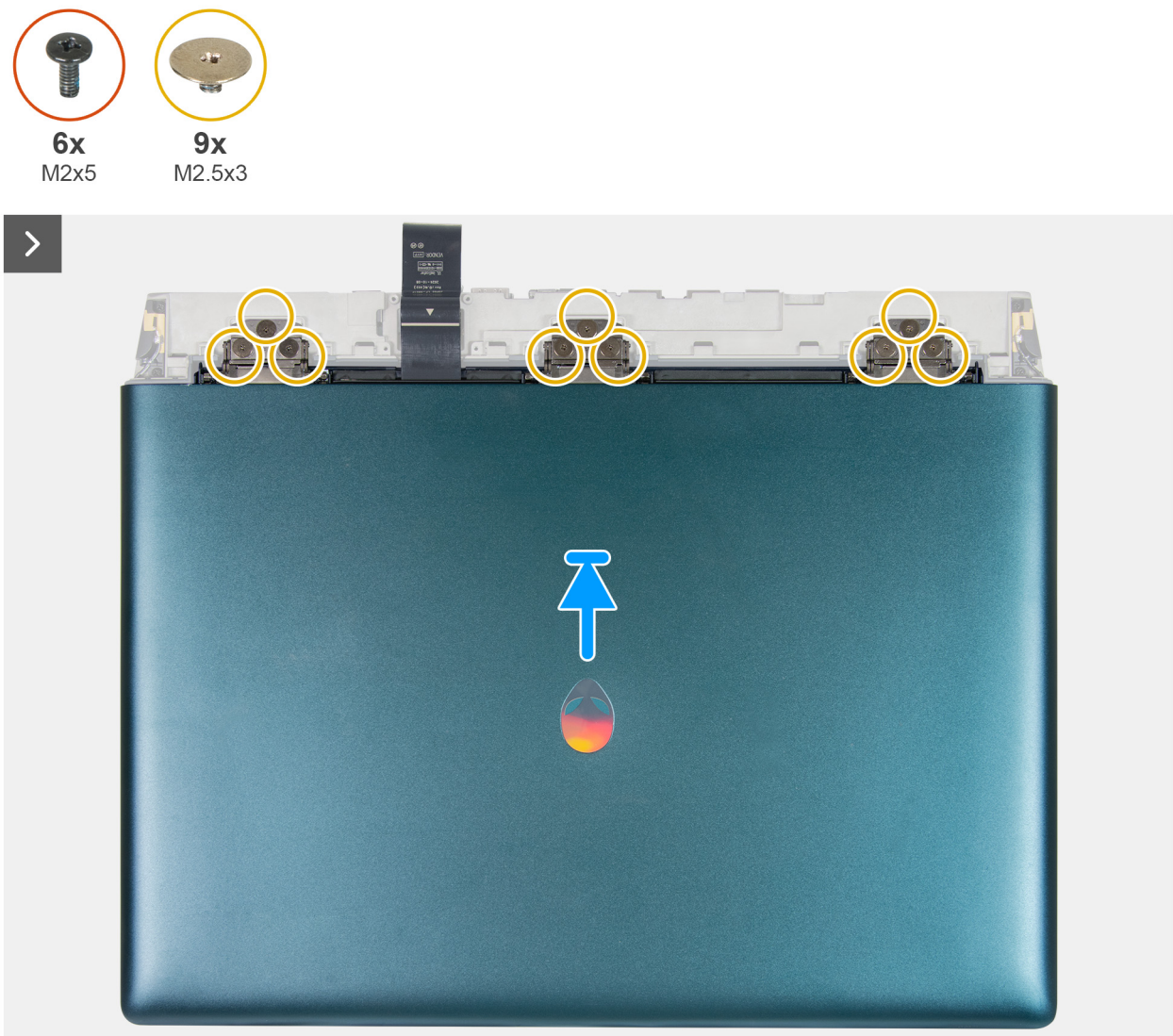
Abbildung 49. Einbauen der Displaybaugruppe
