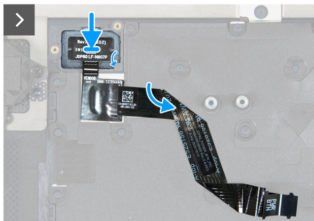
Abbildung 72. Installieren des Netzschalters
