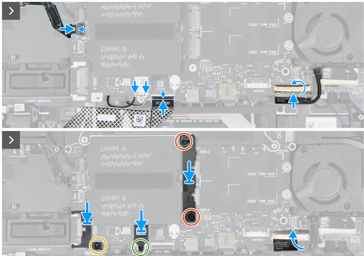
Abbildung 65. Einbauen der Systemplatine
