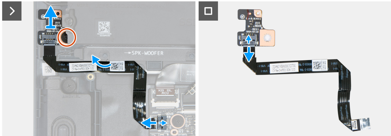
Abbildung 42. Entfernen der Hall-Sensorplatine
