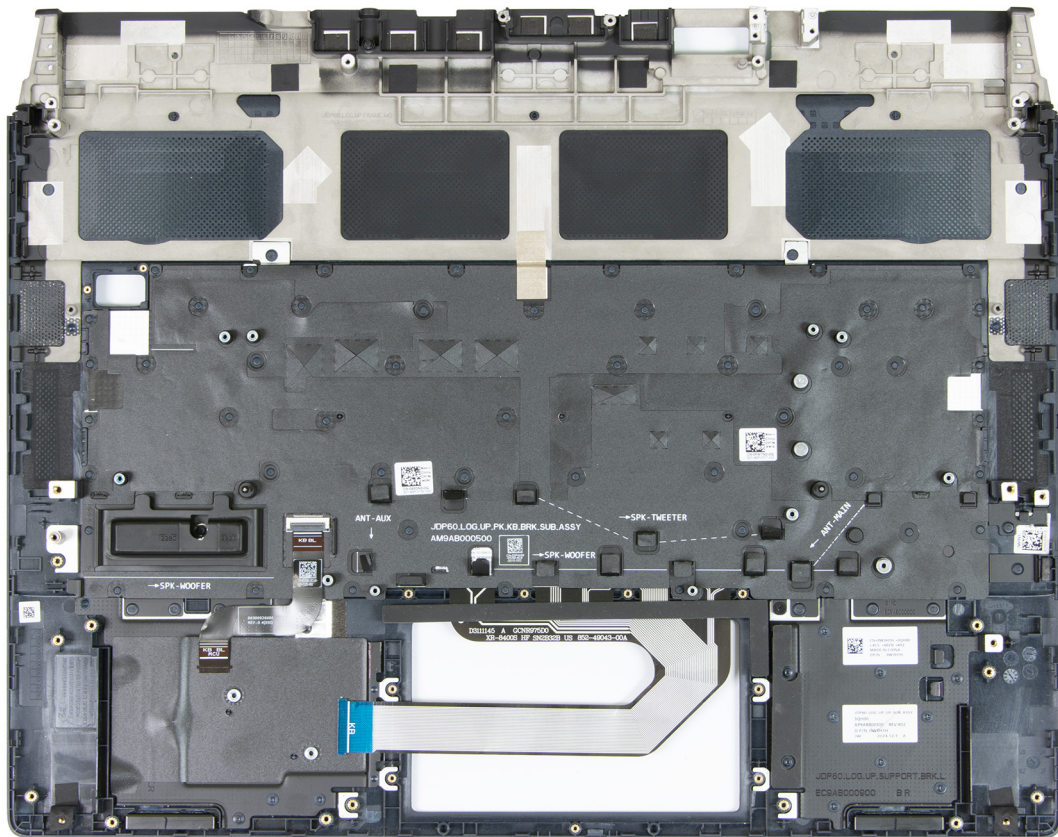
Abbildung 81. Einbauen der Handauflagen-Tastatur-Baugruppe
