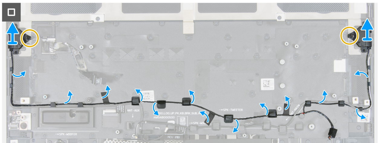
Abbildung 78. Entfernen der Hochtöner
