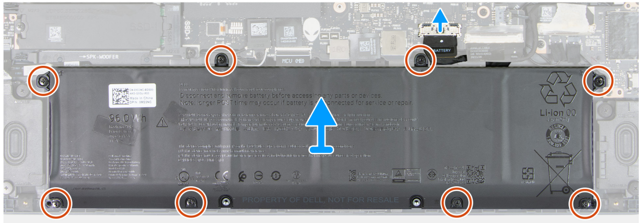
Abbildung 16. Entfernen des Akkus
