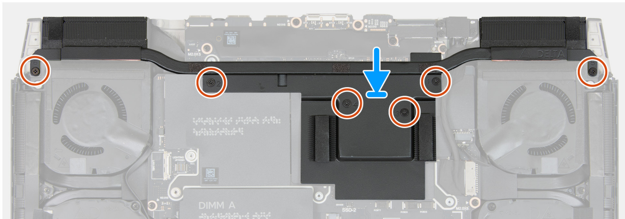
Abbildung 45. Installieren des VR-Kühlkörpers
