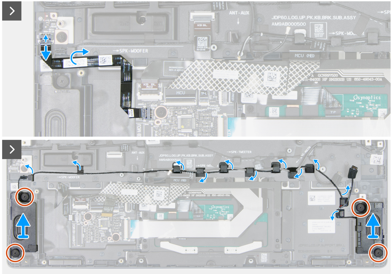
Abbildung 77. Entfernen der Woofer
