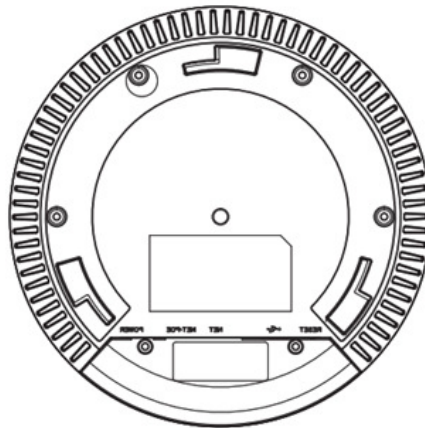
GWN7610/GWN7600 Ports
