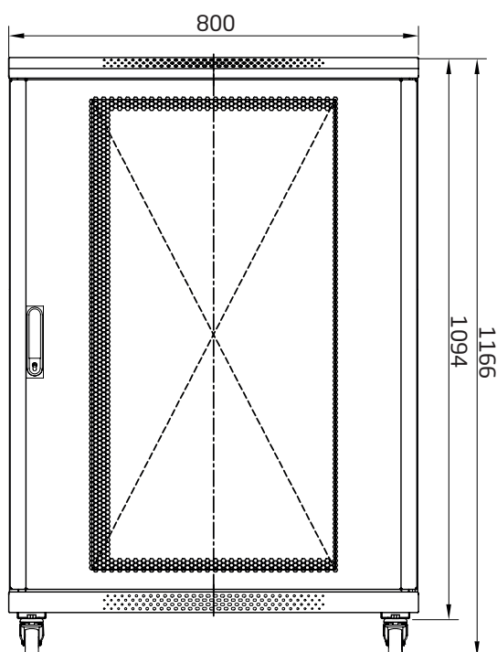
Hinteransicht
