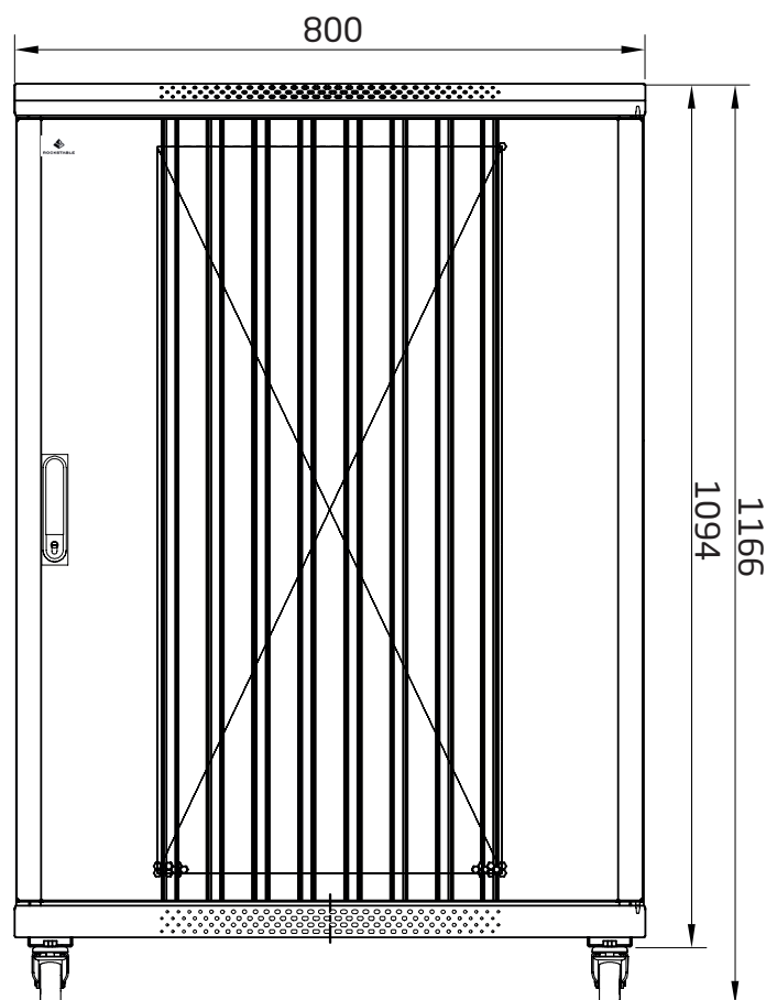
Vorderansicht
