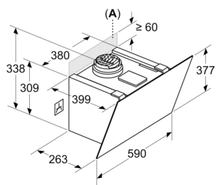
Maße in mm Gerät im Umluftbetrieb ohne Abluftkanal
