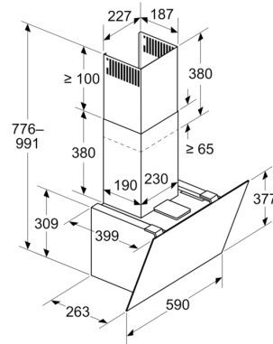
Maße in mm Gerät im Umluftbetrieb
