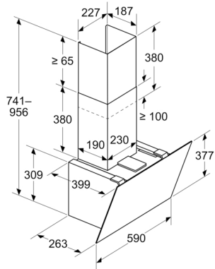
Maße in mm Gerät im Abluftbetrieb
