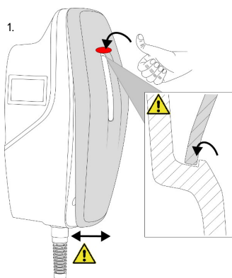
Ilustr. 21: Zakładanie pokrywy przedniej - 1
