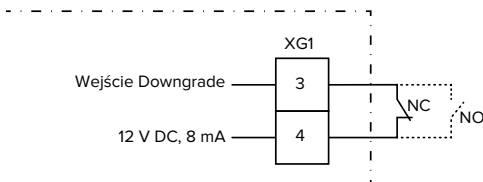
Ilustr. 17: Schemat obwodu: podłączenie zewnętrznego styku przełączającego (ustawienie standardowe: NO)
