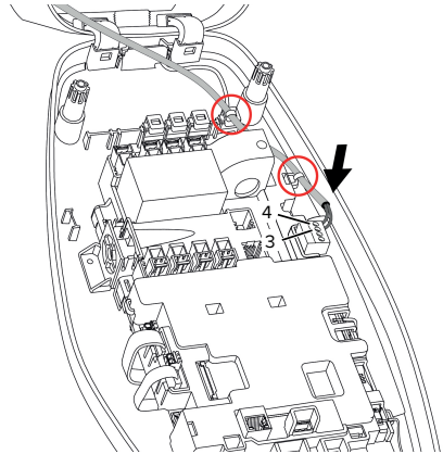
Abb. 16: Anschluss Downgrade-Eingang
