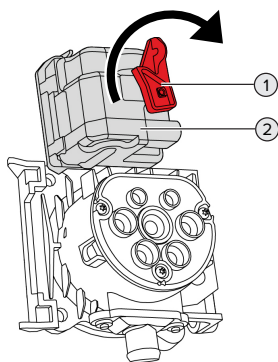
Fig. 25: Desbloquear el conector de carga manualmente
