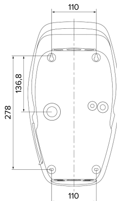
Fig. 8: Borrmått [mm]
