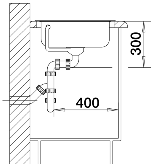
Seitenansicht
