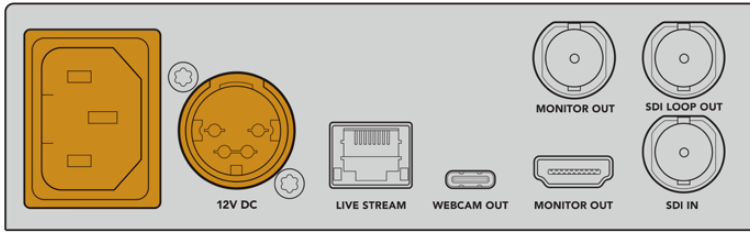
Web Presenter HD, IEC kablosu veya 12V DC güç girişi kullanılarak çalıştırılabilir.
