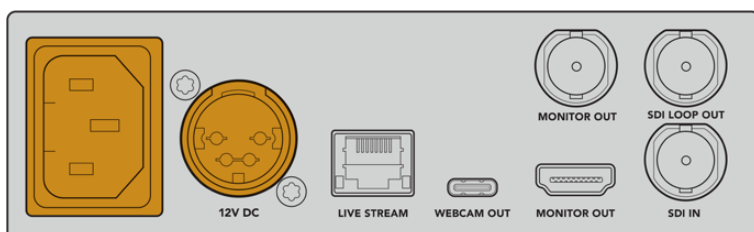
Web Presenter HD si alimenta tramite l'ingresso IEC o 12V DC
