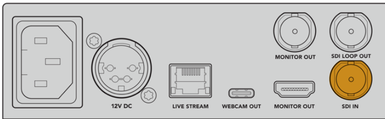
Blackmagic Web Presenter'inizin SDI girişine video sinyali bağlayın
