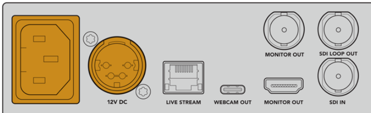
Der Web Presenter HD kann wahlweise über den IEC- oder einen der 12V-DC-Stromeingänge mit Strom versorgt werden
