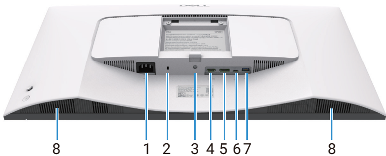
Abbildung 4. Unteransicht des Monitors
