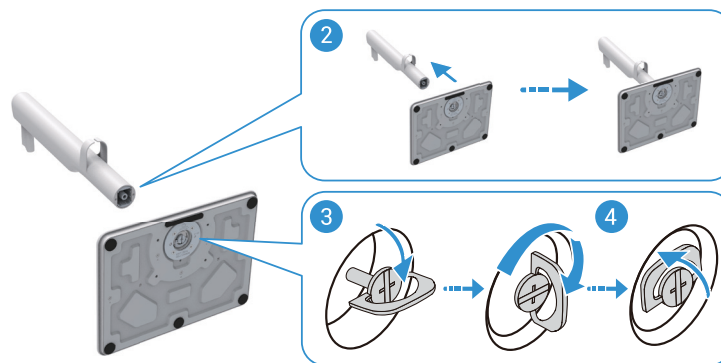
Abbildung 14. Installieren Sie den Ständer und den Standfuß
