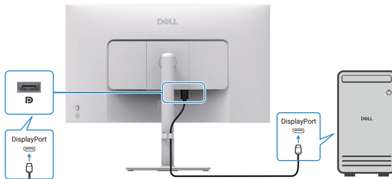
Abbildung 23. Anschließen des DisplayPort-Kabels
