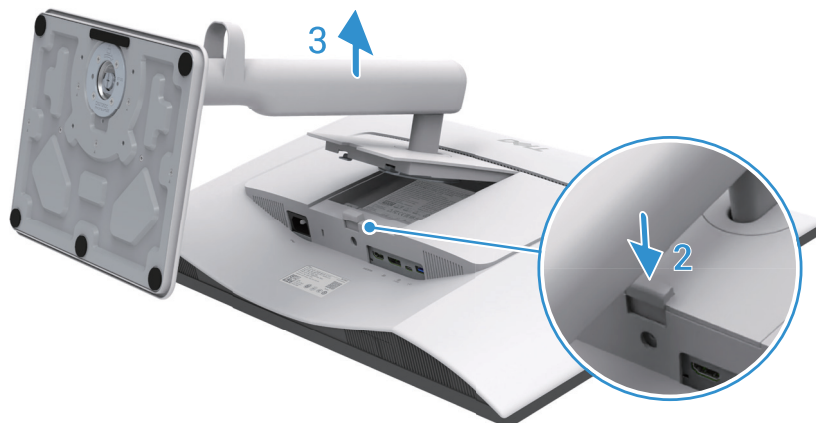
Abbildung 27. Entfernen des Monitorständers
