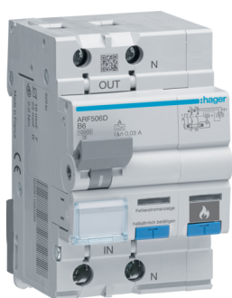
ARF506D
