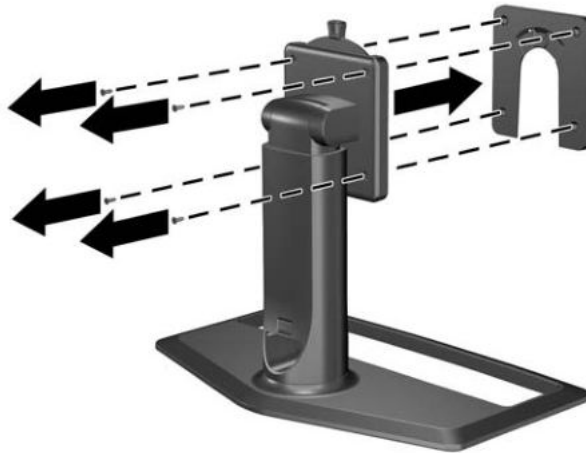
Abbildung 3-11 Abnehmen der HP Schnellverriegelung vom Standfuß
