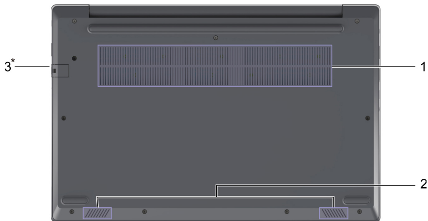
Rysunek 8. Widok z dołu—modele 14-calowe
