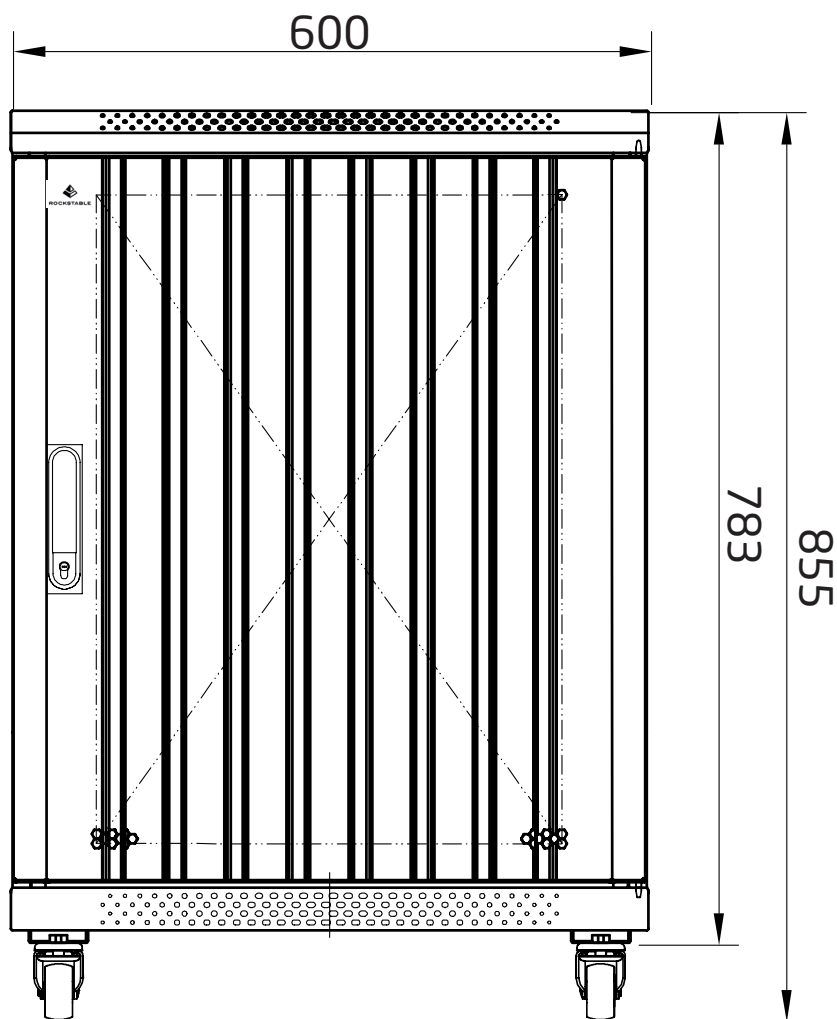
Vorderansicht
