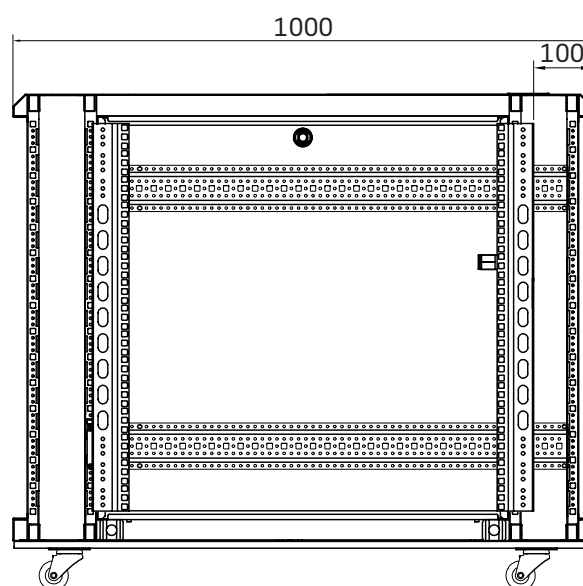
Seiteninnenansicht
