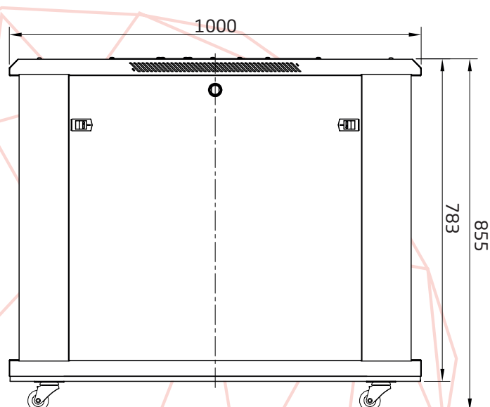
Seitenansicht
