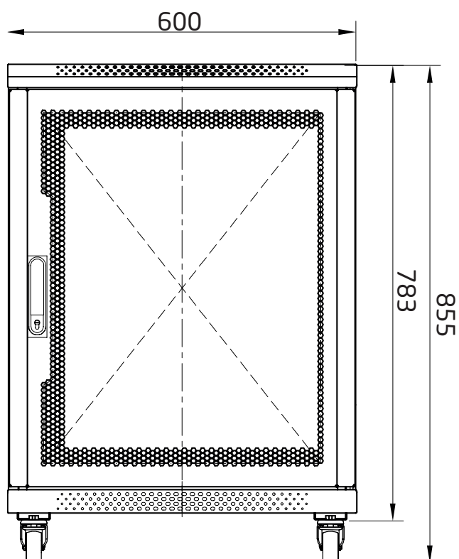
Hinteransicht
