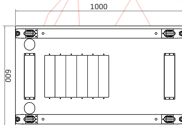
Boden
