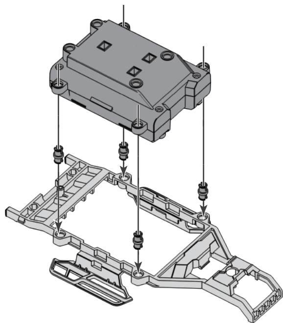
Verbinder / Latch C1 4x
