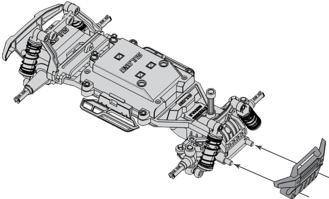
Stoßfänger / Bumper F4-1 1x
