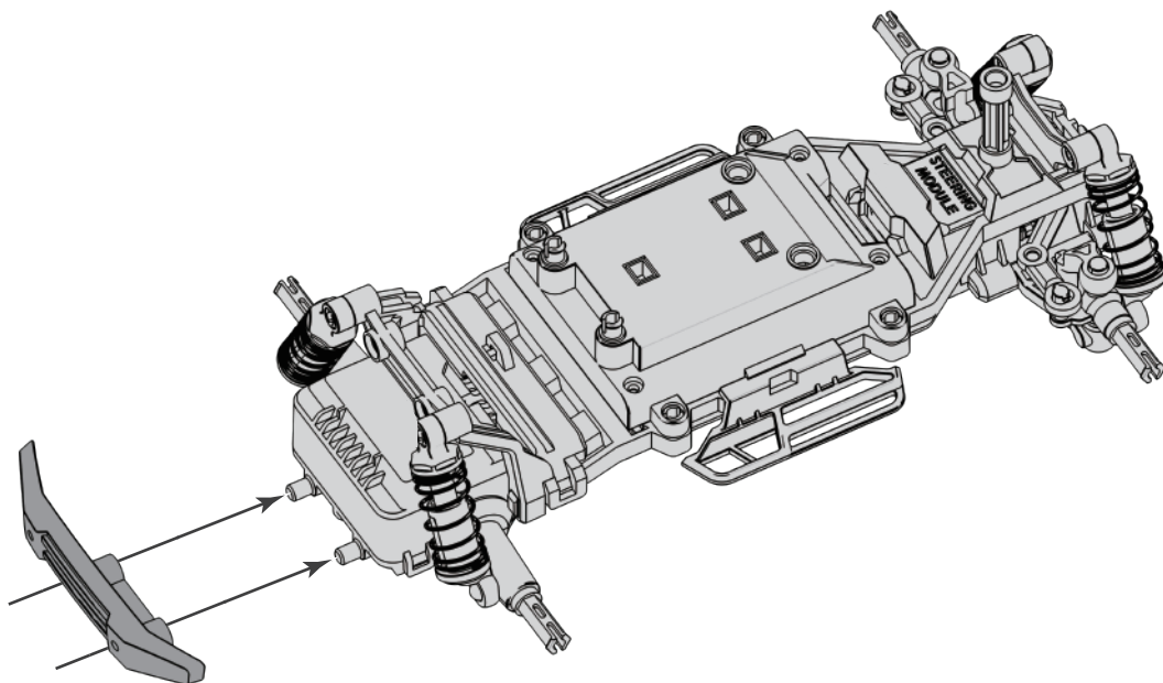
Hinterer Stoßfänger / Rear Bumper F4-2 1x
